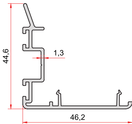
KOD-CODE TEORİK AĞIRLIK THEORETICAL WEIGHT SS-404-13 0,468 Kg/m
