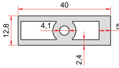
KOD-CODE TEORİK AĞIRLIK THEORETICAL WEIGHT 1493 0,807 Kg/m
