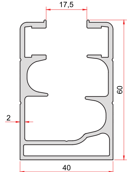
KOD-CODE TEORİK AĞIRLIK 2293 THEORETICAL WEIGHT 1,393 Kg/m
