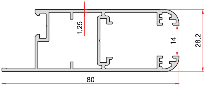
KOD-CODE TEORİK AĞIRLIK THEORETICAL WEIGHT 7026 0,880 Kg/m
