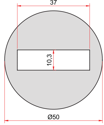
KOD-CODE TEORİK AĞIRLIK THEORETICAL WEIGHT 1863 4,271 Kg/m
