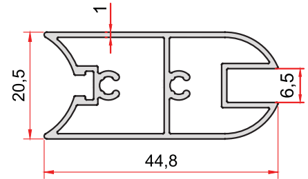
KOD-CODE TEORİK AĞIRLIK THEORETICAL WEIGHT 1772 0,518 Kg/m
