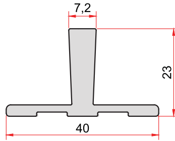
KOD-CODE TEORİK AĞIRLIK 1473 0,618 Kg/m THEORETICAL WEIGHT
