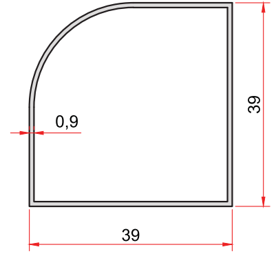
KOD-CODE TEORİK AĞIRLIK THEORETICAL WEIGHT 1437 0,351 Kg/m
