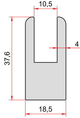
KOD-CODE TEORİK AĞIRLIK 5025 THEORETICAL WEIGHT 1,280 Kg/m
