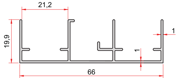
KOD-CODE TEORİK AĞIRLIK THEORETICAL WEIGHT 1453 0,451 Kg/m
