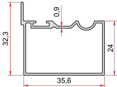
KOD-CODE TEORİK AĞIRLIK 2300 0,343 Kg/m THEORETICAL WEIGHT
