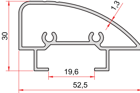
KOD-CODE TEORİK AĞIRLIK 1773 THEORETICAL WEIGHT 0,613 Kg/m
