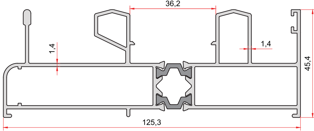
KOD-CODE TEORİK AĞIRLIK SS-101-14 THEORETICAL WEIGHT 2,054 Kg/m
