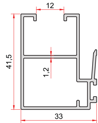
KOD-CODE TEORİK AĞIRLIK 1005 THEORETICAL WEIGHT 0,575 Kg/m
