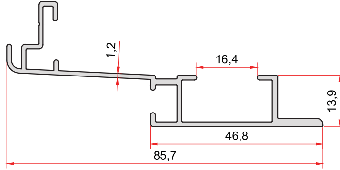
KOD-CODE TEORİK AĞIRLIK THEORETICAL WEIGHT 1080 0,600 Kg/m
