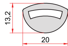
KOD-CODE TEORİK AĞIRLIK THEORETICAL WEIGHT 1410 0,424 Kg/m
