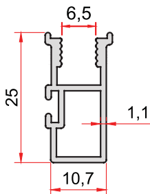
KOD-CODE TEORİK AĞIRLIK THEORETICAL WEIGHT 1783 0,248 Kg/m
