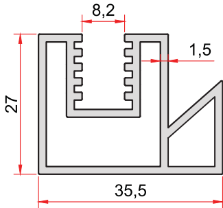
KOD-CODE TEORİK AĞIRLIK 2603 0,732 Kg/m THEORETICAL WEIGHT
