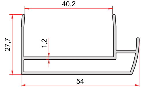
KOD-CODE TEORİK AĞIRLIK THEORETICAL WEIGHT 2392 0,532 Kg/m
