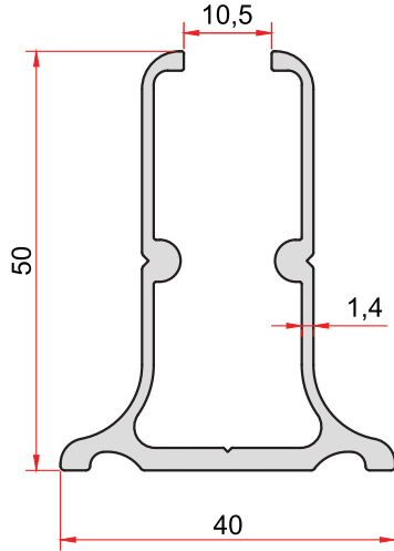
KOD-CODE TEORİK AĞIRLIK THEORETICAL WEIGHT 5039 0,756 Kg/m
