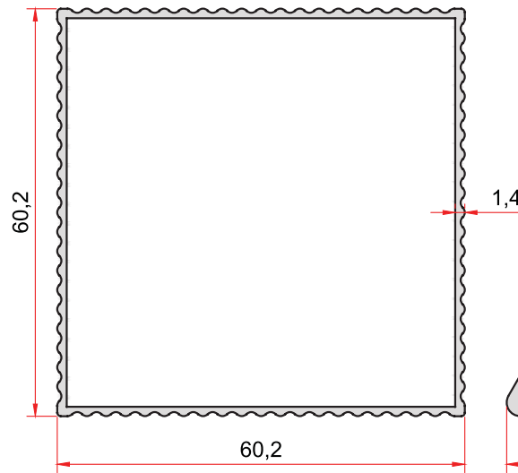
KOD-CODE TEORİK AĞIRLIK 4015 THEORETICAL WEIGHT 0,702 Kg/m
