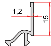
KOD-CODE TEORİK AĞIRLIK THEORETICAL WEIGHT 1206 0,119 Kg/m
