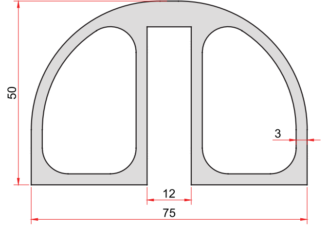
KOD-CODE TEORİK AĞIRLIK THEORETICAL WEIGHT 1878 2,695 Kg/m
