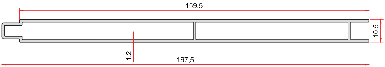
KOD-CODE TEORİK AĞIRLIK THEORETICAL WEIGHT 1203 1,164 Kg/m
