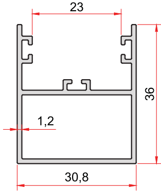
KOD-CODE TEORİK AĞIRLIK 2386 THEORETICAL WEIGHT 0,480 Kg/m
