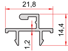
KOD-CODE TEORİK AĞIRLIK 1037 THEORETICAL WEIGHT 0,178 Kg/m
