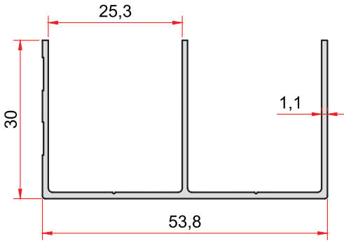
KOD-CODE TEORİK AĞIRLIK THEORETICAL WEIGHT 1401 0,416 Kg/m
