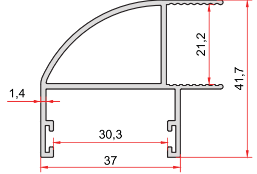
KOD-CODE TEORİK AĞIRLIK 2668 THEORETICAL WEIGHT 0,621 Kg/m
