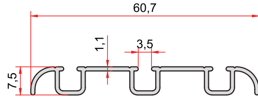
KOD-CODE TEORİK AĞIRLIK THEORETICAL WEIGHT 2697 0,324 Kg/m
