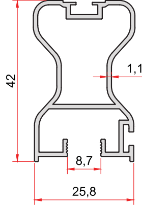
KOD-CODE TEORİK AĞIRLIK THEORETICAL WEIGHT 1365 0,516 Kg/m
