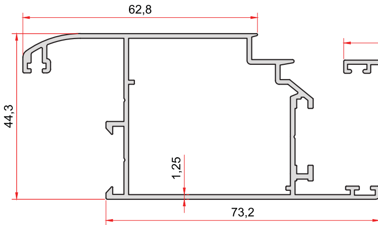
KOD-CODE TEORİK AĞIRLIK THEORETICAL WEIGHT 1130 0,961 Kg/m
