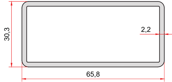
KOD-CODE TEORİK AĞIRLIK THEORETICAL WEIGHT 1972 1,069 Kg/m
