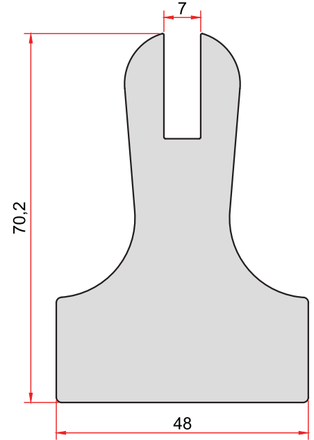
KOD-CODE TEORİK AĞIRLIK 5046 THEORETICAL WEIGHT 5,054 Kg/m
