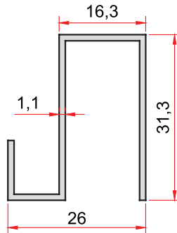
KOD-CODE TEORİK AĞIRLIK 1366 0,300 Kg/m THEORETICAL WEIGHT
