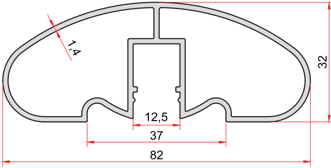
KOD-CODE TEORİK AĞIRLIK THEORETICAL WEIGHT 1998 0,939 Kg/m
