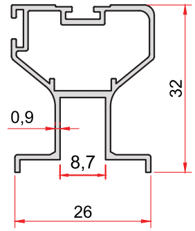
KOD-CODE TEORİK AĞIRLIK THEORETICAL WEIGHT 1380 0,362 Kg/m
