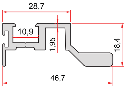
KOD-CODE TEORİK AĞIRLIK 1368 0,637 Kg/m THEORETICAL WEIGHT
