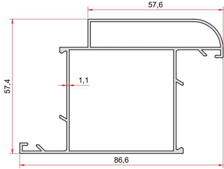
KOD-CODE 805 TEORİK AĞIRLIK THEORETICAL WEIGHT 0,983 Kg/m
