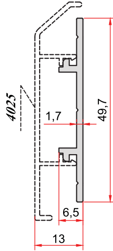
KOD-CODE TEORİK AĞIRLIK 4024 THEORETICAL WEIGHT 0,286 Kg/m
