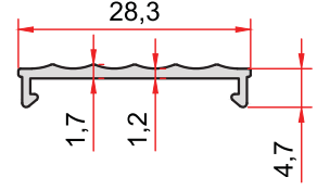
KOD-CODE 2696 TEORİK AĞIRLIK 0,125 THEORETICAL WEIGHT Kg/m
