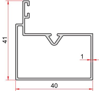
KOD-CODE TEORİK AĞIRLIK THEORETICAL WEIGHT 2296 0,448 Kg/m
