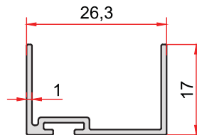
KOD-CODE TEORİK AĞIRLIK 2758 THEORETICAL WEIGHT 0,180 Kg/m
