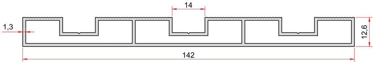
KOD-CODE TEORİK AĞIRLIK THEORETICAL WEIGHT 2383 1,247 Kg/m
