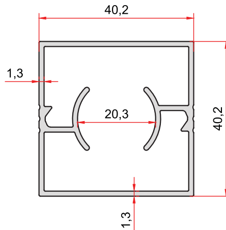
KOD-CODE TEORİK AĞIRLIK 2725 THEORETICAL WEIGHT 0,748 Kg/m
