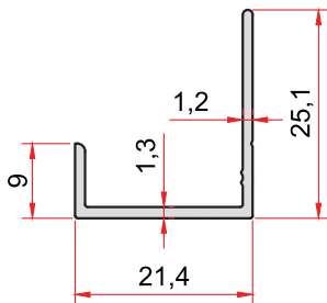
KOD-CODE TEORİK AĞIRLIK 1377 0,178 Kg/m THEORETICAL WEIGHT
