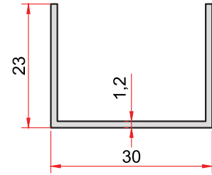
KOD-CODE TEORİK AĞIRLIK THEORETICAL WEIGHT 85 0,238 Kg/m
