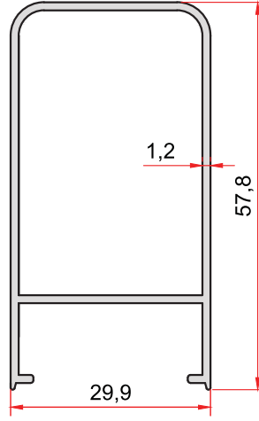
KOD-CODE TEORİK AĞIRLIK THEORETICAL WEIGHT 875 0,551 Kg/m
