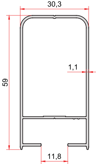
KOD-CODE 769 TEORİK AĞIRLIK 0,543 Kg/m THEORETICAL WEIGHT
