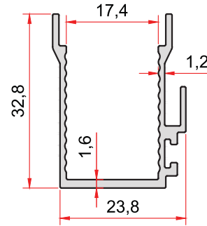
KOD-CODE TEORİK AĞIRLIK 2387 THEORETICAL WEIGHT 0,340 Kg/m
