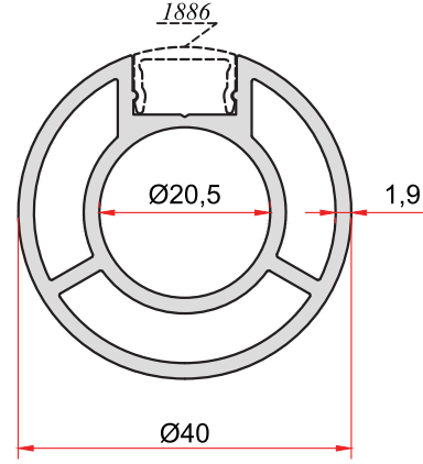
KOD-CODE TEORİK AĞIRLIK THEORETICAL WEIGHT 1990 1,047 Kg/m
