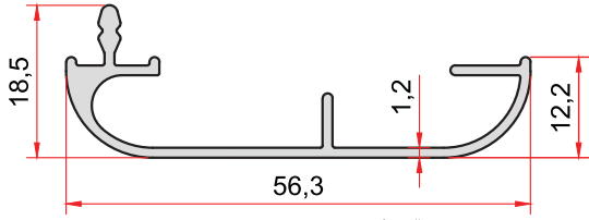
KOD-CODE TEORİK AĞIRLIK 1038 0,373 Kg/m THEORETICAL WEIGHT
