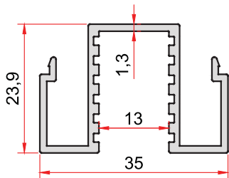
KOD-CODE TEORİK AĞIRLIK THEORETICAL WEIGHT 796 0,440 Kg/m
