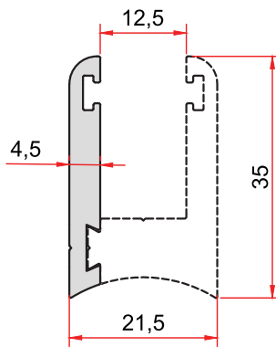
KOD-CODE TEORİK AĞIRLIK 5057 THEORETICAL WEIGHT 0,342 Kg/m
