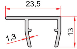
KOD-CODE 1028 TEORİK AĞIRLIK THEORETICAL WEIGHT 0,171 Kg/m
