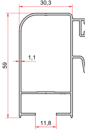
KOD-CODE 770 TEORİK AĞIRLIK 0,643 Kg/m THEORETICAL WEIGHT
