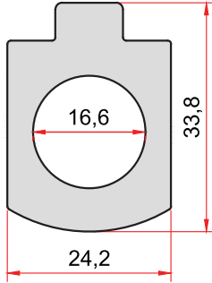
KOD-CODE TEORİK AĞIRLIK THEORETICAL WEIGHT 1855 1,337 Kg/m
