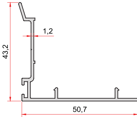
KOD-CODE TEORİK AĞIRLIK 809 THEORETICAL WEIGHT 0,370 Kg/m
