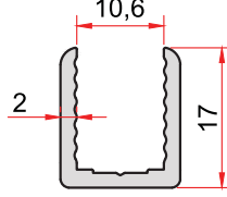
KOD-CODE TEORİK AĞIRLIK 5002 THEORETICAL WEIGHT 0,221 Kg/m
