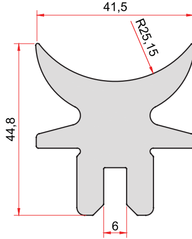
KOD-CODE TEORİK AĞIRLIK 1857 2,403 Kg/m THEORETICAL WEIGHT
