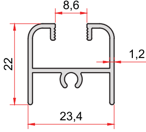
KOD-CODE TEORİK AĞIRLIK THEORETICAL WEIGHT 1361 0,292 Kg/m
