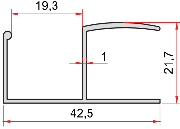
KOD-CODE TEORİK AĞIRLIK 1387 THEORETICAL WEIGHT 0,294 Kg/m
