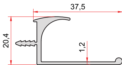
KOD-CODE TEORİK AĞIRLIK THEORETICAL WEIGHT 1498 0,377 Kg/m
