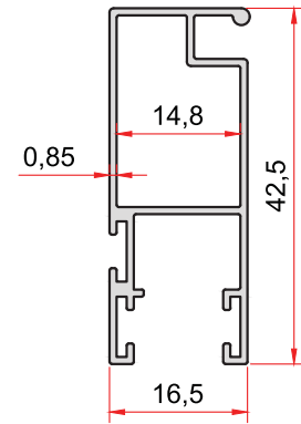
KOD-CODE TEORİK AĞIRLIK THEORETICAL WEIGHT 1310 0,335 Kg/m
