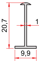
KOD-CODE TEORİK AĞIRLIK THEORETICAL WEIGHT 1432 0,086 Kg/m
