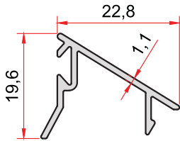
KOD-CODE TEORİK AĞIRLIK 1039 THEORETICAL WEIGHT 0,173 Kg/m
