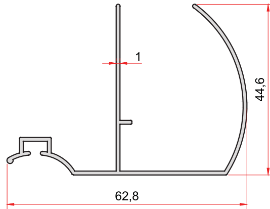
KOD-CODE TEORİK AĞIRLIK 1784 THEORETICAL WEIGHT 0,451 Kg/m
