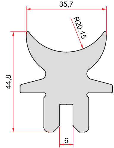
KOD-CODE TEORİK AĞIRLIK 1866 2,400 Kg/m THEORETICAL WEIGHT
