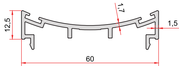
KOD-CODE TEORİK AĞIRLIK THEORETICAL WEIGHT 1243 0,510 Kg/m
