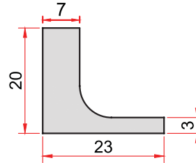
KOD-CODE TEORİK AĞIRLIK THEORETICAL WEIGHT 1414 0,529 Kg/m
