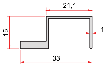
KOD-CODE TEORİK AĞIRLIK 1386 0,246 Kg/m THEORETICAL WEIGHT
