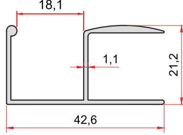
KOD-CODE TEORİK AĞIRLIK 1403 THEORETICAL WEIGHT 0,346 Kg/m
