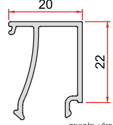
KOD-CODE TEORİK AĞIRLIK THEORETICAL WEIGHT CC-1200-13 0,270 Kg/m
