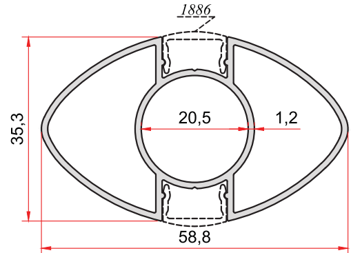
KOD-CODE TEORİK AĞIRLIK 1948 THEORETICAL WEIGHT 0,702 Kg/m
