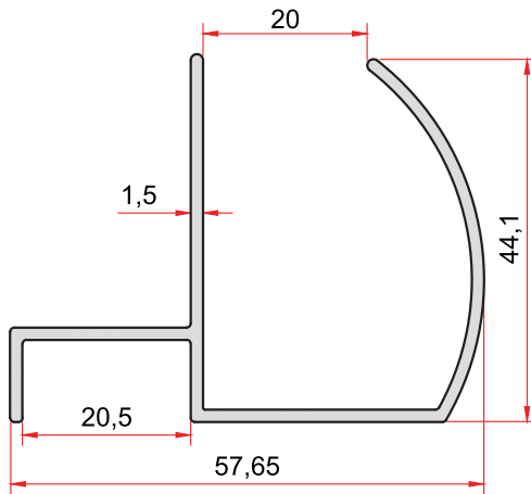
KOD-CODE TEORİK AĞIRLIK 1788 THEORETICAL WEIGHT 0,621 Kg/m
