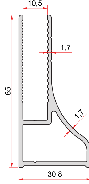
KOD-CODE TEORİK AĞIRLIK THEORETICAL WEIGHT 1914 0,826 Kg/m
