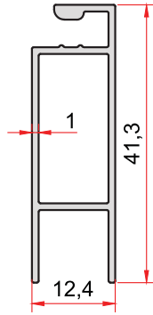
KOD-CODE TEORİK AĞIRLIK THEORETICAL WEIGHT 1027 0,297 Kg/m
