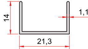
KOD-CODE TEORİK AĞIRLIK THEORETICAL WEIGHT 1388 0,140 Kg/m
