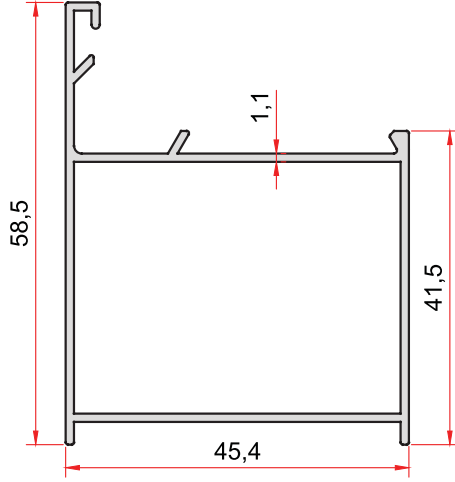
KOD-CODE TEORİK AĞIRLIK THEORETICAL WEIGHT 822 0,599 Kg/m
