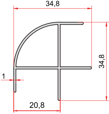
KOD-CODE TEORİK AĞIRLIK THEORETICAL WEIGHT 1390 0,321 Kg/m
