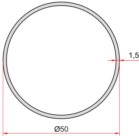
KOD-CODE TEORİK AĞIRLIK THEORETICAL WEIGHT 1884 0,618 Kg/m
