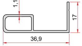
KOD-CODE TEORİK AĞIRLIK 1430 THEORETICAL WEIGHT 0,267 Kg/m
