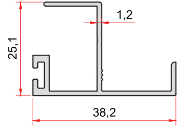
KOD-CODE TEORİK AĞIRLIK 1404 THEORETICAL WEIGHT 0,338 Kg/m
