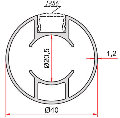
KOD-CODE TEORİK AĞIRLIK 1890 THEORETICAL WEIGHT 0,645 Kg/m
