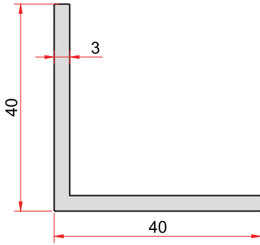
KOD-CODE TEORİK AĞIRLIK THEORETICAL WEIGHT 145 0,623 Kg/m
