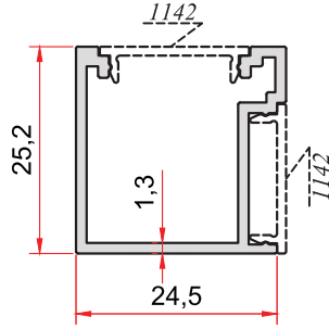
KOD-CODE TEORİK AĞIRLIK 1140 THEORETICAL WEIGHT 0,311 Kg/m
