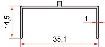
KOD-CODE TEORİK AĞIRLIK THEORETICAL WEIGHT 795 0,178 Kg/m
