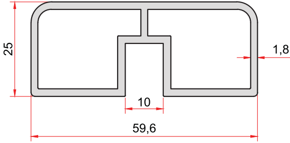
KOD-CODE TEORİK AĞIRLIK THEORETICAL WEIGHT 1876 1,010 Kg/m
