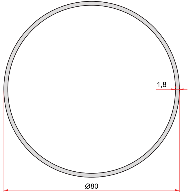
KOD-CODE TEORİK AĞIRLIK THEORETICAL WEIGHT 1936 1,193 Kg/m
