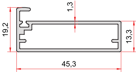
KOD-CODE TEORİK AĞIRLIK 1384 THEORETICAL WEIGHT 0,475 Kg/m
