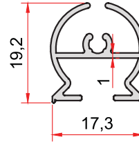
KOD-CODE TEORİK AĞIRLIK THEORETICAL WEIGHT 1753 0,219 Kg/m
