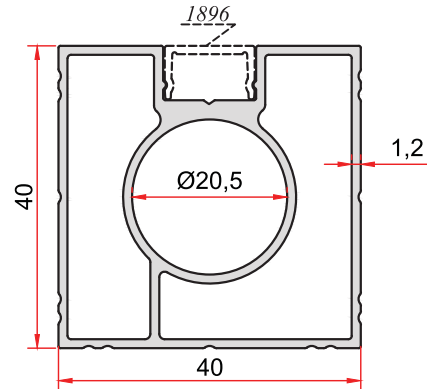
KOD-CODE TEORİK AĞIRLIK 5037 THEORETICAL WEIGHT 0,823 Kg/m
