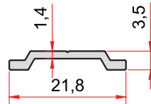
KOD-CODE TEORİK AĞIRLIK 836 THEORETICAL WEIGHT 0,097 Kg/m
