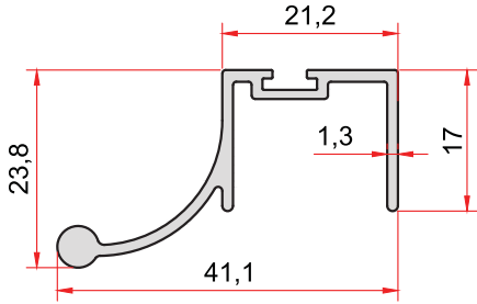
KOD-CODE TEORİK AĞIRLIK 1405 THEORETICAL WEIGHT 0,329 Kg/m
