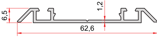
KOD-CODE TEORİK AĞIRLIK THEORETICAL WEIGHT 1423 0,313 Kg/m
