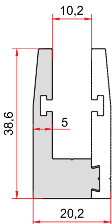
KOD-CODE TEORİK AĞIRLIK 5098 THEORETICAL WEIGHT 0,769 Kg/m
