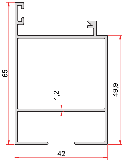
KOD-CODE TEORİK AĞIRLIK THEORETICAL WEIGHT 782 0,788 Kg/m
