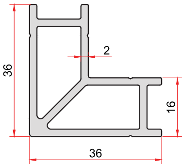
KOD-CODE TEORİK AĞIRLIK THEORETICAL WEIGHT 1160 0,831 Kg/m
