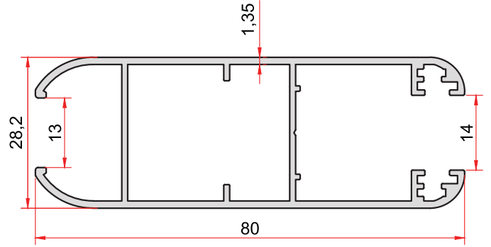
KOD-CODE TEORİK AĞIRLIK THEORETICAL WEIGHT 1136 0,880 Kg/m
