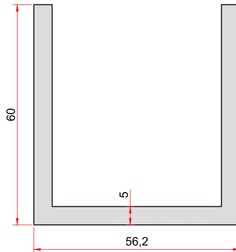
KOD-CODE TEORİK AĞIRLIK THEORETICAL WEIGHT 88 2,244 Kg/m
