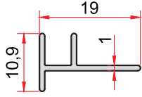
KOD-CODE TEORİK AĞIRLIK THEORETICAL WEIGHT 1503 0,091 Kg/m
