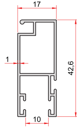
KOD-CODE TEORİK AĞIRLIK THEORETICAL WEIGHT 1066 0,389 Kg/m
