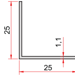
KOD-CODE TEORİK AĞIRLIK THEORETICAL WEIGHT 15 0,146 Kg/m
