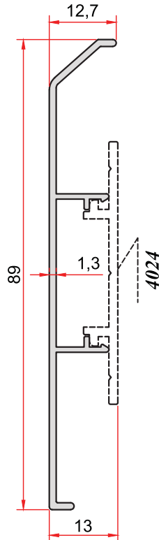
KOD-CODE TEORİK AĞIRLIK 4026 THEORETICAL WEIGHT 0,410 Kg/m
