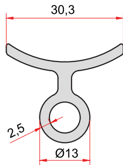
KOD-CODE TEORİK AĞIRLIK THEORETICAL WEIGHT 5071 0,497 Kg/m
