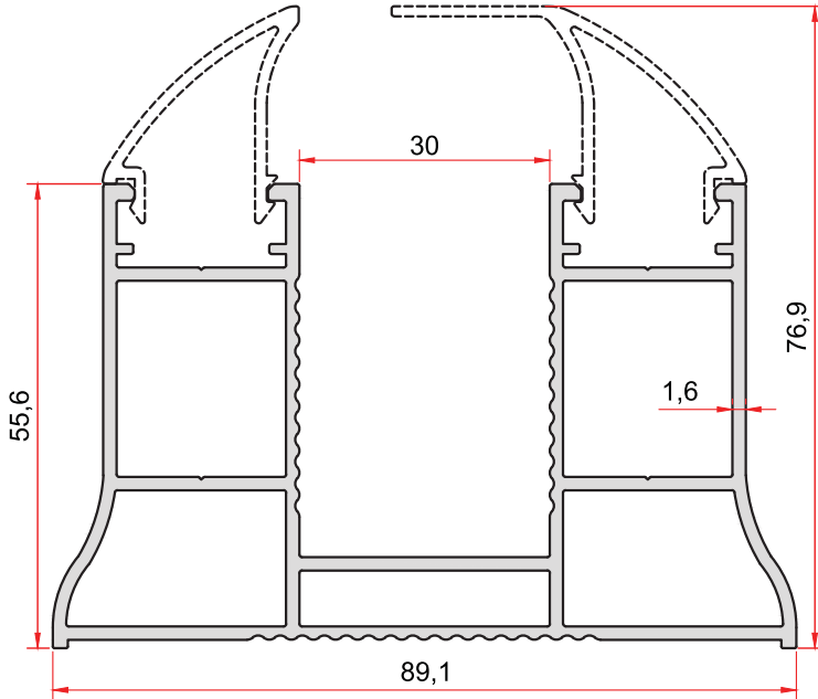
KOD-CODE TEORİK AĞIRLIK THEORETICAL WEIGHT 5017 1,804 Kg/m
