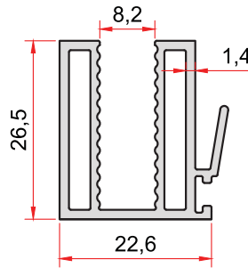
KOD-CODE TEORİK AĞIRLIK 2388 0,507 Kg/m THEORETICAL WEIGHT
