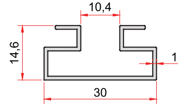
KOD-CODE TEORİK AĞIRLIK THEORETICAL WEIGHT 1389 0,232 Kg/m
