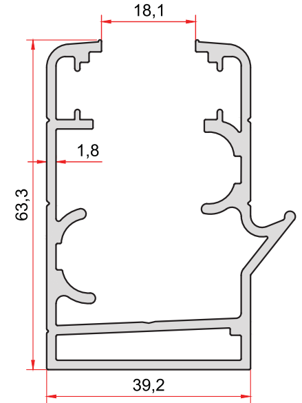
KOD-CODE TEORİK AĞIRLIK THEORETICAL WEIGHT 2653 1,393 Kg/m
