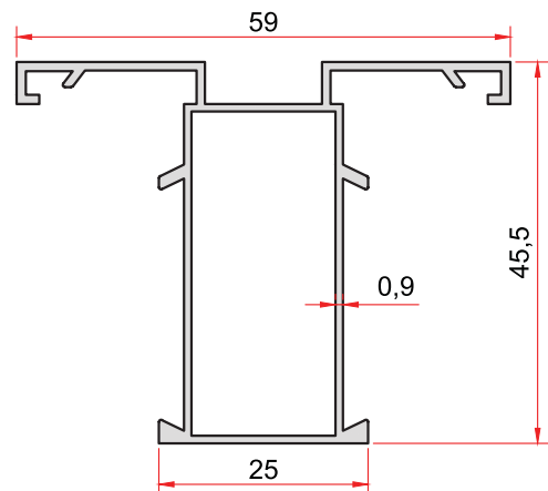
KOD-CODE TEORİK AĞIRLIK THEORETICAL WEIGHT 862 0,537 Kg/m
