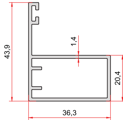
KOD-CODE TEORİK AĞIRLIK 2756 THEORETICAL WEIGHT 0,564 Kg/m
