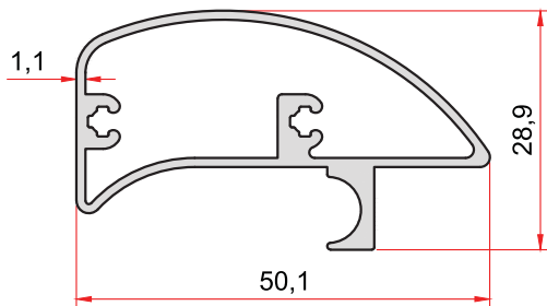
KOD-CODE TEORİK AĞIRLIK 1779 THEORETICAL WEIGHT 0,575 Kg/m
