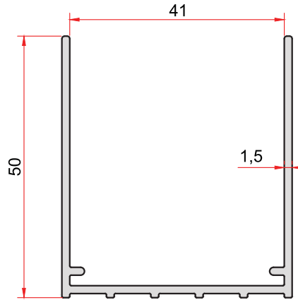
KOD-CODE 2636 TEORİK AĞIRLIK THEORETICAL WEIGHT 0,605 Kg/m
