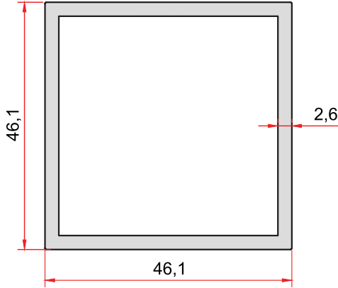
KOD-CODE TEORİK AĞIRLIK THEORETICAL WEIGHT 1965 1,220 Kg/m
