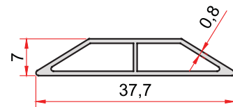
KOD-CODE TEORİK AĞIRLIK 4002 THEORETICAL WEIGHT 0,189 Kg/m
