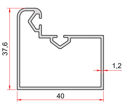
KOD-CODE TEORİK AĞIRLIK THEORETICAL WEIGHT 2294 0,540 Kg/m
