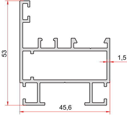
KOD-CODE TEORİK AĞIRLIK THEORETICAL WEIGHT 7033 0,899 Kg/m
