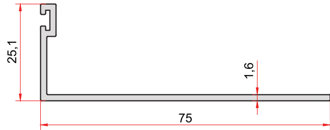
KOD-CODE TEORİK AĞIRLIK THEORETICAL WEIGHT 155 0,454 Kg/m
