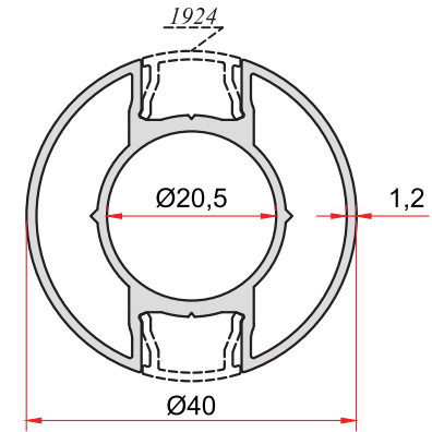
KOD-CODE TEORİK AĞIRLIK 1925 THEORETICAL WEIGHT 0,721 Kg/m
