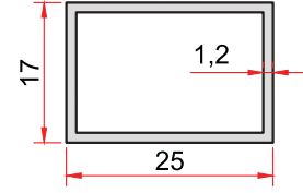
KOD-CODE TEORİK AĞIRLIK 114 THEORETICAL WEIGHT 0,256 Kg/m
