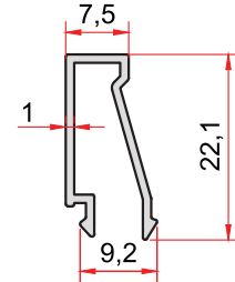
KOD-CODE TEORİK AĞIRLIK THEORETICAL WEIGHT SS-602-10 0,145 Kg/m
