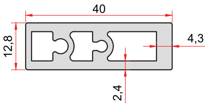
KOD-CODE TEORİK AĞIRLIK THEORETICAL WEIGHT 1499 0,797 Kg/m
