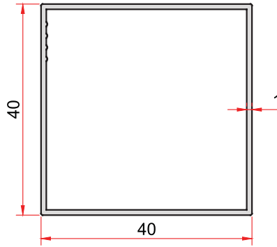
KOD-CODE 773 TEORİK AĞIRLIK 0,421 Kg/m THEORETICAL WEIGHT
