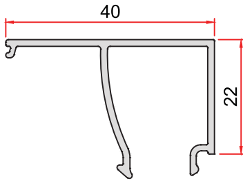
KOD-CODE TEORİK AĞIRLIK THEORETICAL WEIGHT CC-1400-13 0,341 Kg/m
