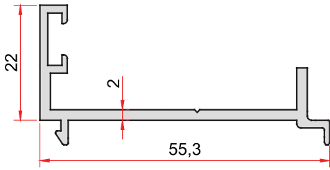
KOD-CODE TEORİK AĞIRLIK THEORETICAL WEIGHT 848 0,502 Kg/m
