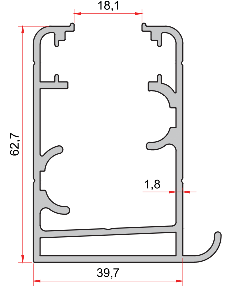
KOD-CODE TEORİK AĞIRLIK THEORETICAL WEIGHT 2450 1,378 Kg/m
