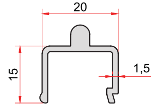
KOD-CODE TEORİK AĞIRLIK THEORETICAL WEIGHT 810 0,262 Kg/m
