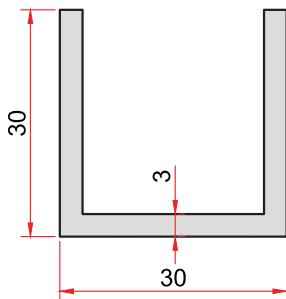
KOD-CODE TEORİK AĞIRLIK THEORETICAL WEIGHT 87 0,680 Kg/m
