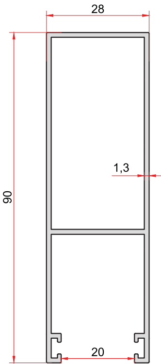
KOD-CODE TEORİK AĞIRLIK 7009 THEORETICAL WEIGHT 0,861 Kg/m
