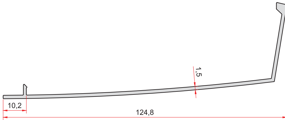
KOD-CODE TEORİK AĞIRLIK THEORETICAL WEIGHT 1996 0,662 Kg/m
