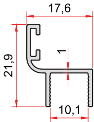
KOD-CODE 2377 TEORİK AĞIRLIK 0,151 THEORETICAL WEIGHT Kg/m
