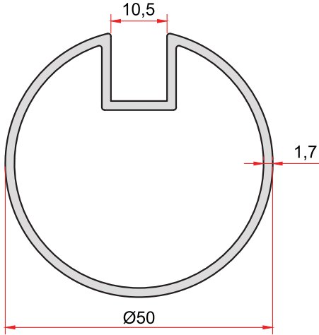
KOD-CODE TEORİK AĞIRLIK THEORETICAL WEIGHT 1929 0,810 Kg/m
