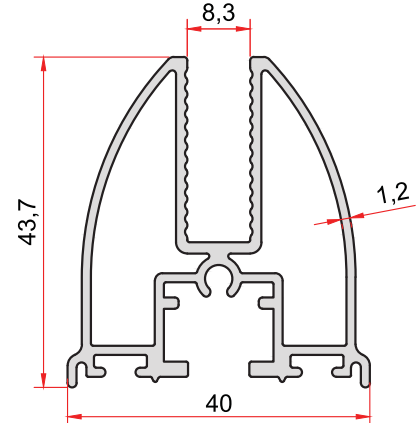
KOD-CODE TEORİK AĞIRLIK THEORETICAL WEIGHT 2637 0,847 Kg/m
