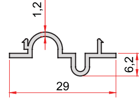
KOD-CODE TEORİK AĞIRLIK 818 THEORETICAL WEIGHT 0,167 Kg/m
