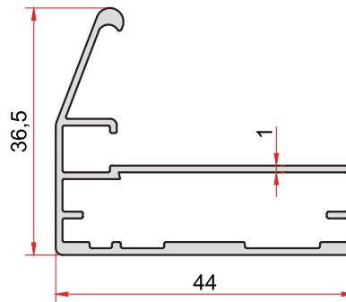
KOD-CODE TEORİK AĞIRLIK 1461 THEORETICAL WEIGHT 0,475 Kg/m
