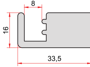
KOD-CODE TEORİK AĞIRLIK 1488 THEORETICAL WEIGHT 1,107 Kg/m
