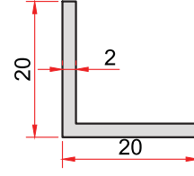
KOD-CODE TEORİK AĞIRLIK THEORETICAL WEIGHT 34 0,205 Kg/m
