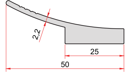
KOD-CODE TEORİK AĞIRLIK THEORETICAL WEIGHT 1471 0,645 Kg/m
