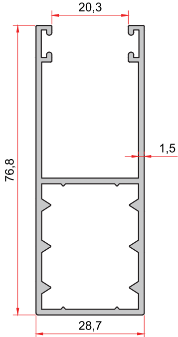
KOD-CODE TEORİK AĞIRLIK THEORETICAL WEIGHT 1075 0,953 Kg/m
