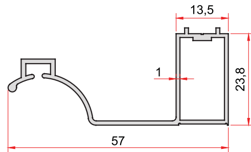
KOD-CODE TEORİK AĞIRLIK 1781 THEORETICAL WEIGHT 0,400 Kg/m
