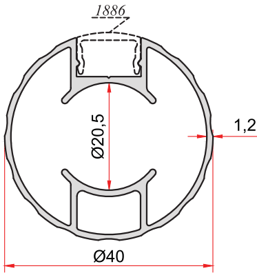
KOD-CODE TEORİK AĞIRLIK 1904 THEORETICAL WEIGHT 0,580 Kg/m
