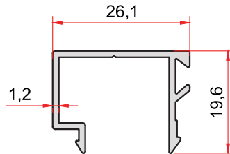
KOD-CODE TEORİK AĞIRLIK 7030 THEORETICAL WEIGHT 0,240 Kg/m
