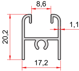
KOD-CODE TEORİK AĞIRLIK THEORETICAL WEIGHT 1395 0,216 Kg/m
