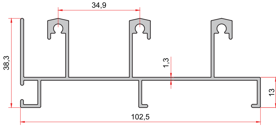
KOD-CODE TEORİK AĞIRLIK THEORETICAL WEIGHT 1078 1,190 Kg/m
