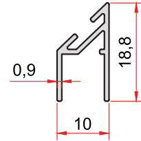
KOD-CODE 2264 TEORİK AĞIRLIK 0,113 THEORETICAL WEIGHT Kg/m
