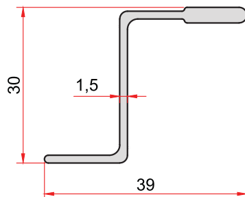
KOD-CODE TEORİK AĞIRLIK THEORETICAL WEIGHT 1308 0,413 Kg/m
