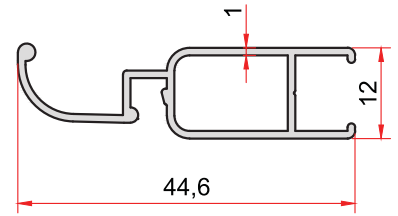
KOD-CODE TEORİK AĞIRLIK THEORETICAL WEIGHT 1303 0,286 Kg/m
