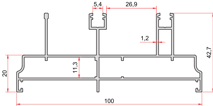
KOD-CODE TEORİK AĞIRLIK THEORETICAL WEIGHT 1139 1,188 Kg/m
