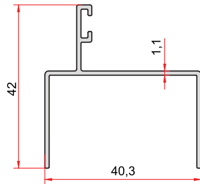
KOD-CODE 2667 TEORİK AĞIRLIK 0,337 THEORETICAL WEIGHT Kg/m
