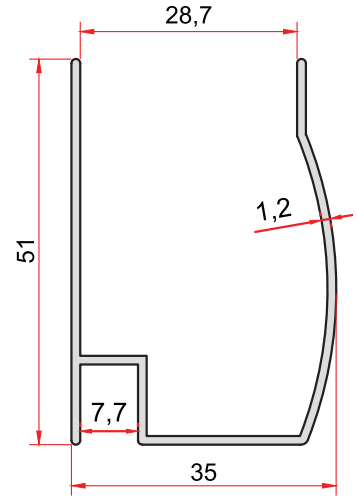
KOD-CODE TEORİK AĞIRLIK 1777 THEORETICAL WEIGHT 0,440 Kg/m
