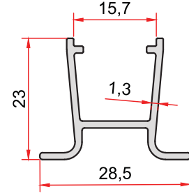
KOD-CODE TEORİK AĞIRLIK SS-501-13 THEORETICAL WEIGHT 0,262 Kg/m
