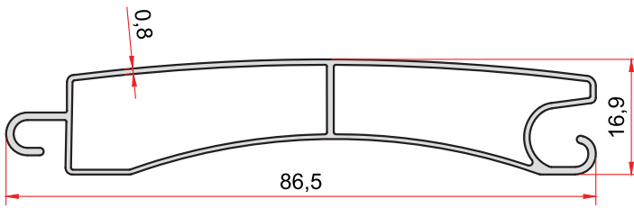
KOD-CODE TEORİK AĞIRLIK THEORETICAL WEIGHT 2310 0,486 Kg/m
