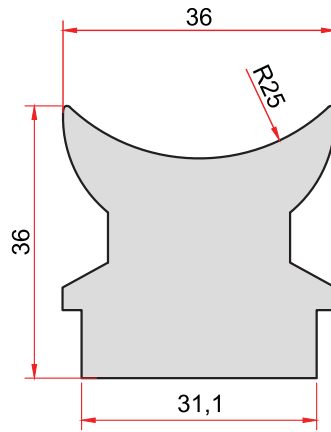
KOD-CODE TEORİK AĞIRLIK 1970 2,549 Kg/m THEORETICAL WEIGHT
