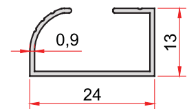
KOD-CODE 779 TEORİK AĞIRLIK 0,143 Kg/m THEORETICAL WEIGHT
