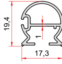
KOD-CODE TEORİK AĞIRLIK THEORETICAL WEIGHT 1752 0,216 Kg/m
