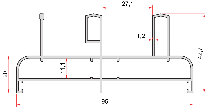
KOD-CODE TEORİK AĞIRLIK THEORETICAL WEIGHT 1134 1,218 Kg/m
