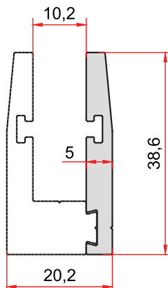
KOD-CODE TEORİK AĞIRLIK 5099 THEORETICAL WEIGHT 0,421 Kg/m
