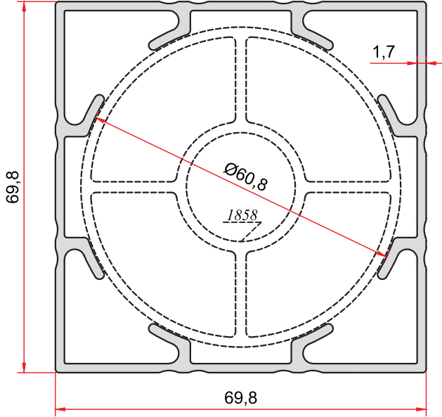
KOD-CODE TEORİK AĞIRLIK THEORETICAL WEIGHT 1898 1,687 Kg/m
