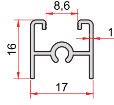
KOD-CODE TEORİK AĞIRLIK THEORETICAL WEIGHT 1399 0,175 Kg/m
