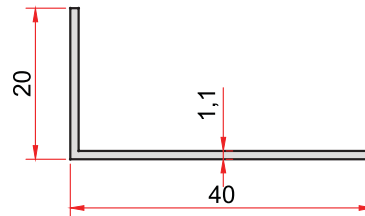
KOD-CODE TEORİK AĞIRLIK THEORETICAL WEIGHT 17 0,176 Kg/m
