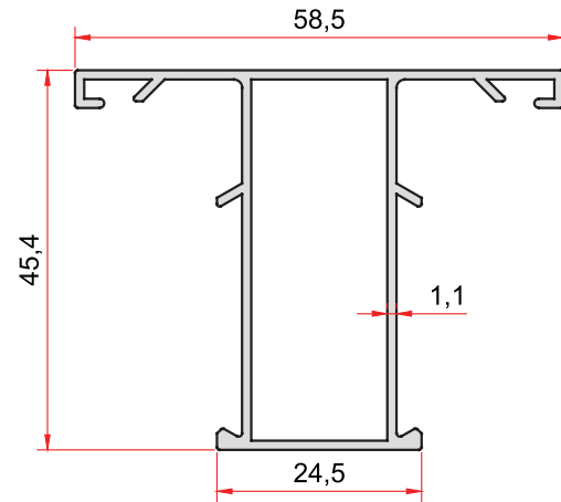
KOD-CODE TEORİK AĞIRLIK THEORETICAL WEIGHT 827 0,594 Kg/m
