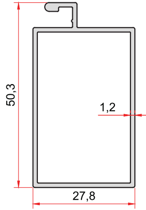
KOD-CODE TEORİK AĞIRLIK THEORETICAL WEIGHT 1010 0,504 Kg/m
