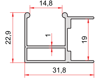
KOD-CODE TEORİK AĞIRLIK 1505 THEORETICAL WEIGHT 0,335 Kg/m
