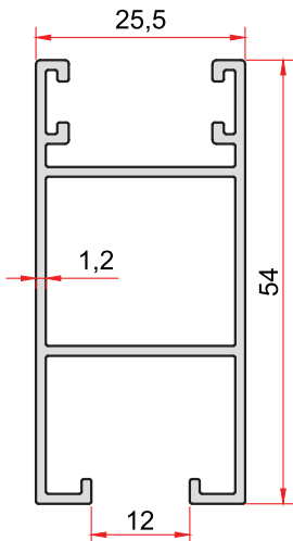
KOD-CODE TEORİK AĞIRLIK 1002 THEORETICAL WEIGHT 0,605 Kg/m
