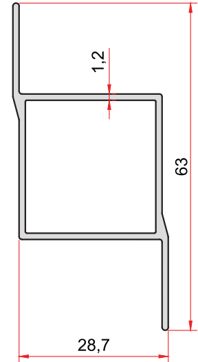
KOD-CODE TEORİK AĞIRLIK THEORETICAL WEIGHT 1018 0,475 Kg/m
