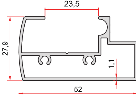
KOD-CODE TEORİK AĞIRLIK 1754 THEORETICAL WEIGHT 0,596 Kg/m
