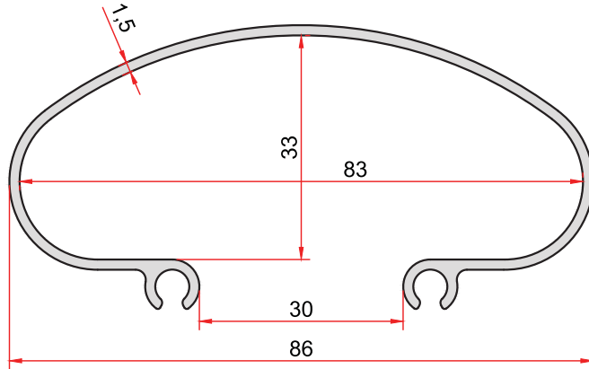
KOD-CODE TEORİK AĞIRLIK THEORETICAL WEIGHT 5062 0,785 Kg/m
