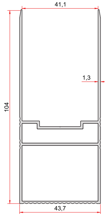
KOD-CODE TEORİK AĞIRLIK THEORETICAL WEIGHT 2663 1,150 Kg/m
