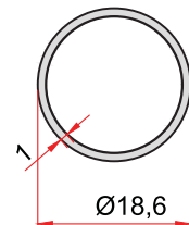
KOD-CODE 5076 TEORİK AĞIRLIK THEORETICAL WEIGHT 0,149 Kg/m
