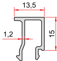
KOD-CODE TEORİK AĞIRLIK THEORETICAL WEIGHT 1205 0,181 Kg/m
