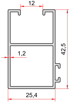
KOD-CODE TEORİK AĞIRLIK 1011 THEORETICAL WEIGHT 0,495 Kg/m
