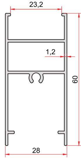
KOD-CODE TEORİK AĞIRLIK THEORETICAL WEIGHT 876 0,610 Kg/m
