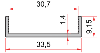
KOD-CODE TEORİK AĞIRLIK 2449 0,181 Kg/m THEORETICAL WEIGHT
