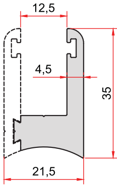
KOD-CODE TEORİK AĞIRLIK 5056 THEORETICAL WEIGHT 0,697 Kg/m
