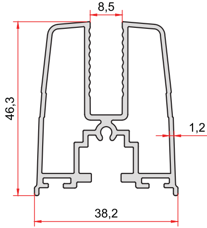
KOD-CODE TEORİK AĞIRLIK 2753 THEORETICAL WEIGHT 0,888 Kg/m
