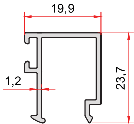
KOD-CODE TEORİK AĞIRLIK 7029 THEORETICAL WEIGHT 0,246 Kg/m
