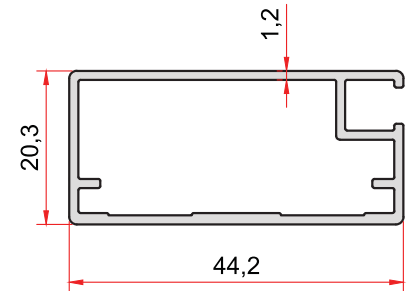
KOD-CODE TEORİK AĞIRLIK 1462 THEORETICAL WEIGHT 0,467 Kg/m
