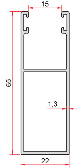
KOD-CODE TEORİK AĞIRLIK 1070 THEORETICAL WEIGHT 0,623 Kg/m
