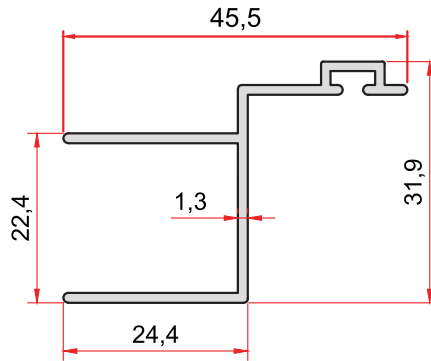
KOD-CODE TEORİK AĞIRLIK THEORETICAL WEIGHT 1782 0,364 Kg/m
