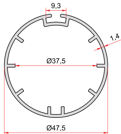
KOD-CODE 2210 TEORİK AĞIRLIK THEORETICAL WEIGHT 0,697 Kg/m
