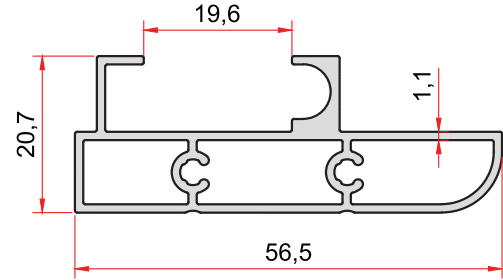
KOD-CODE TEORİK AĞIRLIK 1786 THEORETICAL WEIGHT 0,594 Kg/m
