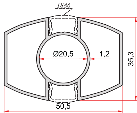
KOD-CODE TEORİK AĞIRLIK 1949 THEORETICAL WEIGHT 0,710 Kg/m
