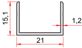
KOD-CODE TEORİK AĞIRLIK THEORETICAL WEIGHT 1481 0,156 Kg/m
