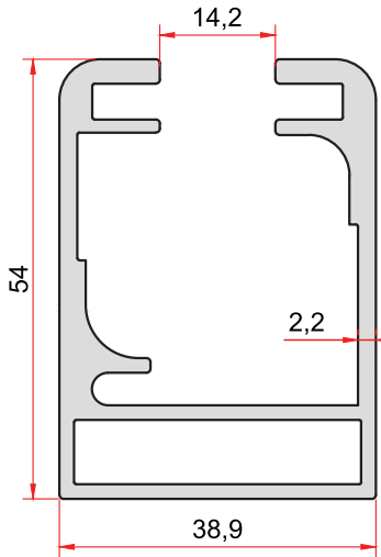
KOD-CODE 2270 TEORİK AĞIRLIK THEORETICAL WEIGHT 1,404 Kg/m
