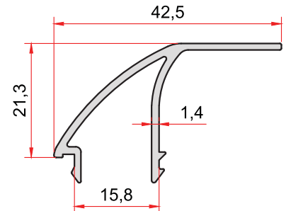
KOD-CODE TEORİK AĞIRLIK THEORETICAL WEIGHT 5018 0,313 Kg/m
