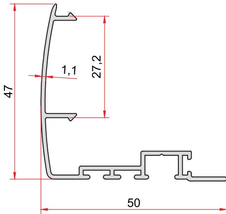
KOD-CODE TEORİK AĞIRLIK THEORETICAL WEIGHT ASS-4513-11 0,415 Kg/m
