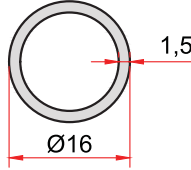
KOD-CODE 1885 TEORİK AĞIRLIK THEORETICAL WEIGHT 0,184 Kg/m
