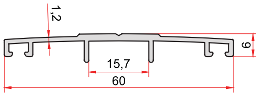
KOD-CODE TEORİK AĞIRLIK 1063 THEORETICAL WEIGHT 0,321 Kg/m
