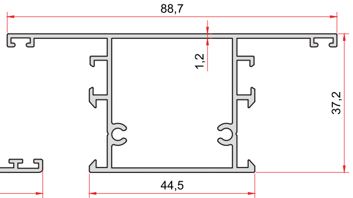
KOD-CODE TEORİK AĞIRLIK THEORETICAL WEIGHT 1132 0,859 Kg/m
