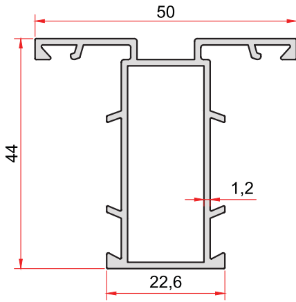
KOD-CODE TEORİK AĞIRLIK THEORETICAL WEIGHT 1083 0,626 Kg/m
