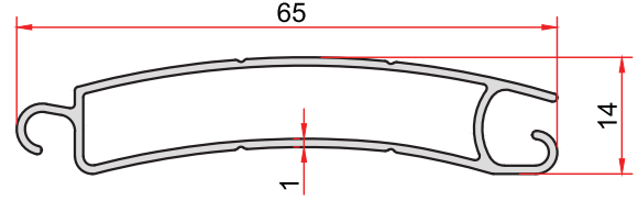
KOD-CODE TEORİK AĞIRLIK THEORETICAL WEIGHT 2316 0,410 Kg/m
