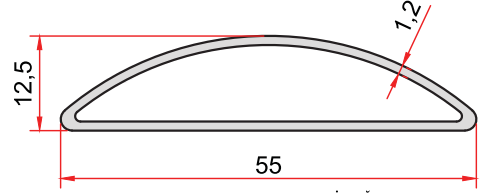
KOD-CODE TEORİK AĞIRLIK THEORETICAL WEIGHT 5058 0,371 Kg/m
