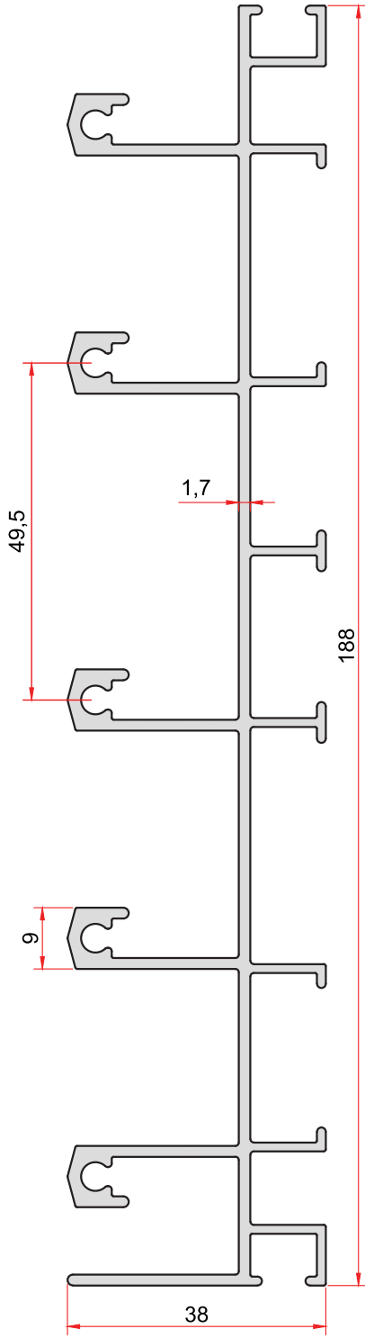
KOD-CODE TEORİK AĞIRLIK THEORETICAL WEIGHT 1000 2,387 Kg/m
