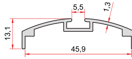
KOD-CODE TEORİK AĞIRLIK 863 THEORETICAL WEIGHT 0,310 Kg/m
