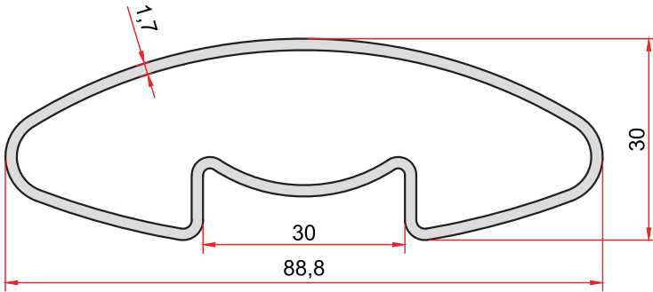
KOD-CODE TEORİK AĞIRLIK THEORETICAL WEIGHT 5041 0,977 Kg/m
