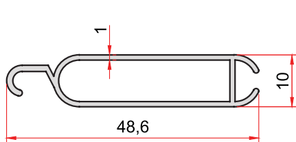
KOD-CODE TEORİK AĞIRLIK THEORETICAL WEIGHT 2305 0,297 Kg/m
