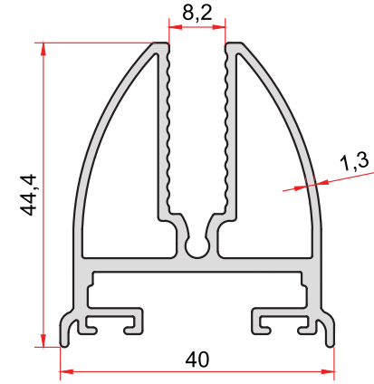
KOD-CODE TEORİK AĞIRLIK THEORETICAL WEIGHT 2292 0,923 Kg/m
