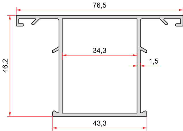
KOD-CODE TEORİK AĞIRLIK THEORETICAL WEIGHT 907 0,921 Kg/m
