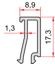
KOD-CODE TEORİK AĞIRLIK THEORETICAL WEIGHT SS-303-13 0,179 Kg/m
