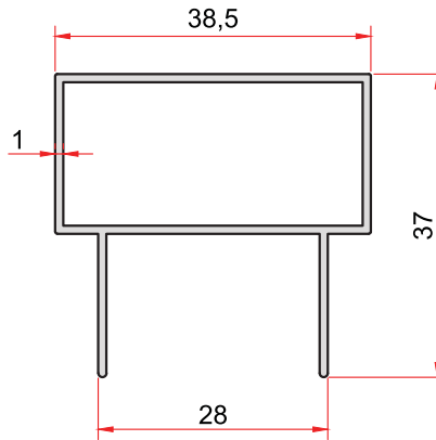
KOD-CODE TEORİK AĞIRLIK THEORETICAL WEIGHT 1305 0,397 Kg/m
