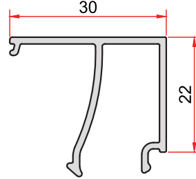
KOD-CODE TEORİK AĞIRLIK THEORETICAL WEIGHT CC-1300-13 0,305 Kg/m
