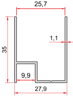
KOD-CODE TEORİK AĞIRLIK 1758 THEORETICAL WEIGHT 0,313 Kg/m
