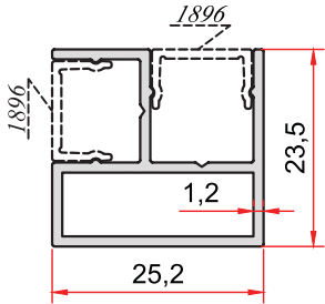
KOD-CODE TEORİK AĞIRLIK 5063 THEORETICAL WEIGHT 0,335 Kg/m
