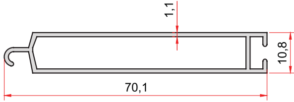
KOD-CODE TEORİK AĞIRLIK THEORETICAL WEIGHT 2303 0,470 Kg/m
