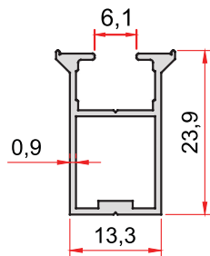
KOD-CODE TEORİK AĞIRLIK THEORETICAL WEIGHT 1763 0,224 Kg/m
