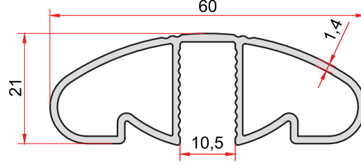
KOD-CODE TEORİK AĞIRLIK THEORETICAL WEIGHT 5067 0,629 Kg/m
