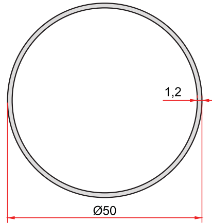
KOD-CODE TEORİK AĞIRLIK THEORETICAL WEIGHT 5059 0,496 Kg/m
