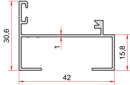
KOD-CODE TEORİK AĞIRLIK THEORETICAL WEIGHT 781 0,348 Kg/m
