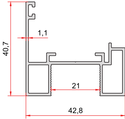
KOD-CODE TEORİK AĞIRLIK 2732 THEORETICAL WEIGHT 0,529 Kg/m
