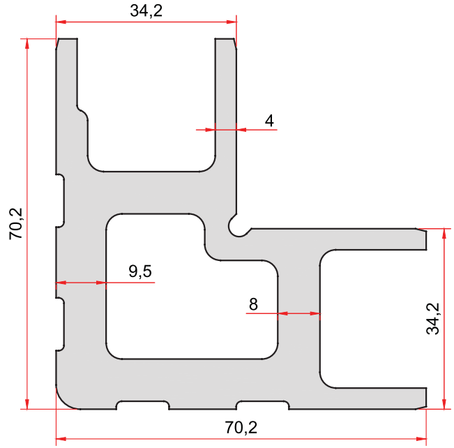
KOD-CODE TEORİK AĞIRLIK THEORETICAL WEIGHT 843 4,417 Kg/m
