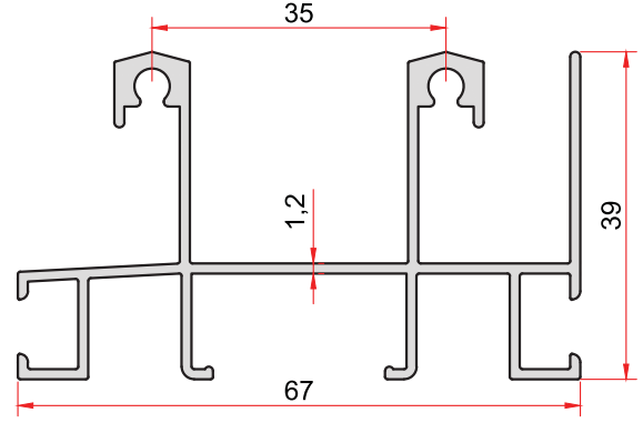
KOD-CODE TEORİK AĞIRLIK 1081 THEORETICAL WEIGHT 0,888 Kg/m
