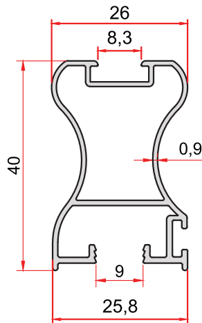
KOD-CODE TEORİK AĞIRLIK THEORETICAL WEIGHT 1452 0,408 Kg/m
