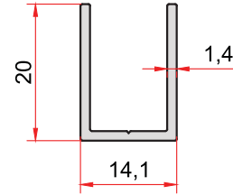
KOD-CODE TEORİK AĞIRLIK THEORETICAL WEIGHT 7035 0,194 Kg/m
