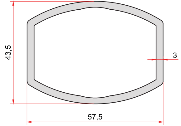
KOD-CODE TEORİK AĞIRLIK THEORETICAL WEIGHT 5038 1,306 Kg/m
