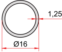
KOD-CODE 1916 TEORİK AĞIRLIK THEORETICAL WEIGHT 0,157 Kg/m
