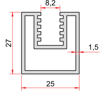
KOD-CODE TEORİK AĞIRLIK 2602 0,575 Kg/m THEORETICAL WEIGHT
