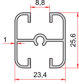
KOD-CODE TEORİK AĞIRLIK THEORETICAL WEIGHT 1362 0,316 Kg/m
