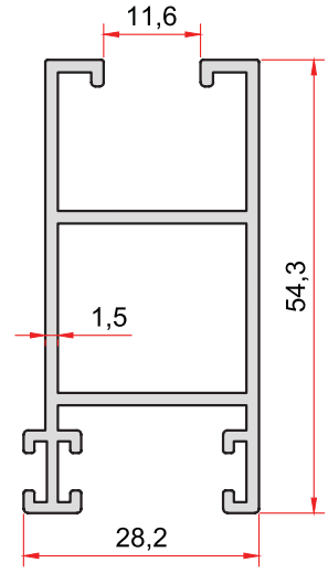
KOD-CODE TEORİK AĞIRLIK 1071 THEORETICAL WEIGHT 0,762 Kg/m
