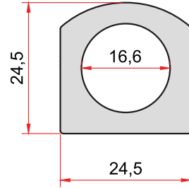
KOD-CODE TEORİK AĞIRLIK THEORETICAL WEIGHT 1941 0,940 Kg/m
