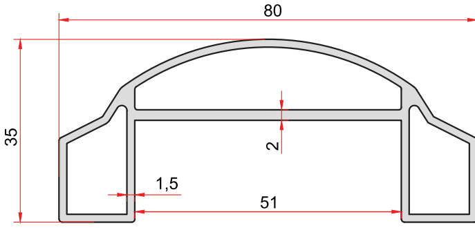
KOD-CODE TEORİK AĞIRLIK THEORETICAL WEIGHT 148 1,075 Kg/m
