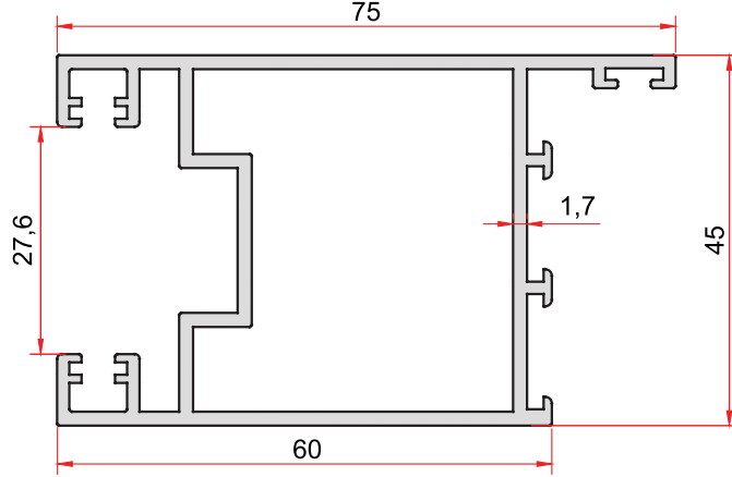
KOD-CODE TEORİK AĞIRLIK 807 THEORETICAL WEIGHT 1,280 Kg/m
