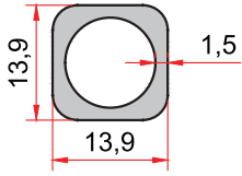
KOD-CODE 1906 TEORİK AĞIRLIK 0,248 Kg/m THEORETICAL WEIGHT
