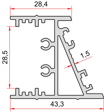
KOD-CODE TEORİK AĞIRLIK 2633 THEORETICAL WEIGHT 0,843 Kg/m
