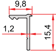
KOD-CODE TEORİK AĞIRLIK THEORETICAL WEIGHT AO-1032-13 0,078 Kg/m
