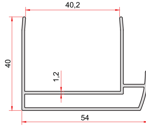
KOD-CODE TEORİK AĞIRLIK THEORETICAL WEIGHT 2619 0,610 Kg/m
