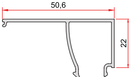
KOD-CODE TEORİK AĞIRLIK THEORETICAL WEIGHT CC-1506-13 0,378 Kg/m
