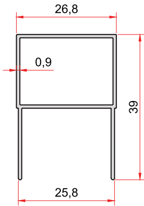
KOD-CODE TEORİK AĞIRLIK THEORETICAL WEIGHT 1307 0,311 Kg/m
