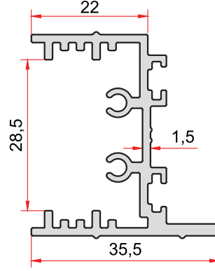
KOD-CODE TEORİK AĞIRLIK 2632 THEORETICAL WEIGHT 0,656 Kg/m
