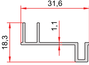
KOD-CODE TEORİK AĞIRLIK THEORETICAL WEIGHT 1789 0,207 Kg/m
