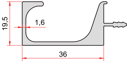
KOD-CODE TEORİK AĞIRLIK 1486 THEORETICAL WEIGHT 0,583 Kg/m
