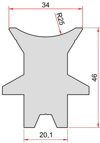
KOD-CODE TEORİK AĞIRLIK 1967 2,738 Kg/m THEORETICAL WEIGHT
