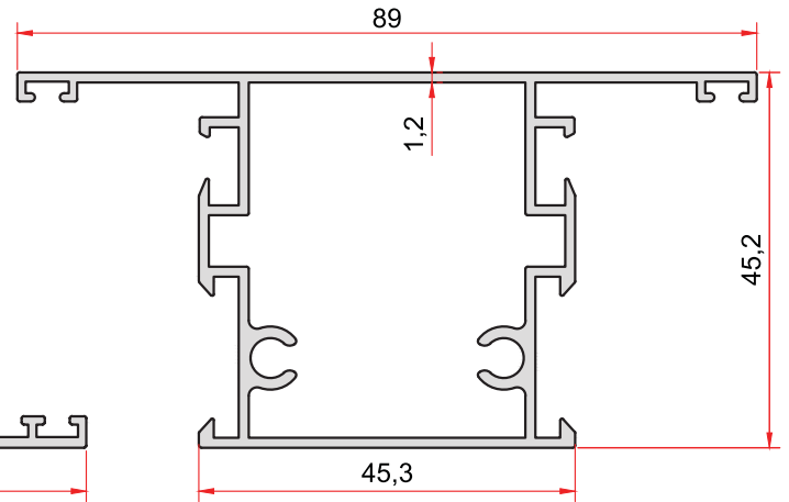
KOD-CODE TEORİK AĞIRLIK THEORETICAL WEIGHT 1153 0,994 Kg/m
