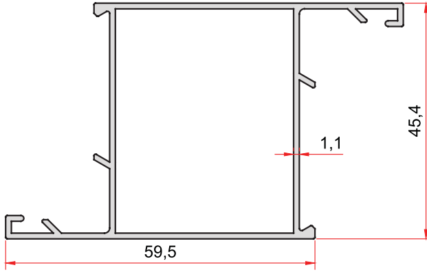
KOD-CODE TEORİK AĞIRLIK THEORETICAL WEIGHT 824 0,702 Kg/m
