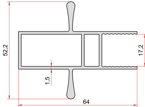
KOD-CODE TEORİK AĞIRLIK 2385 THEORETICAL WEIGHT 0,956 Kg/m
