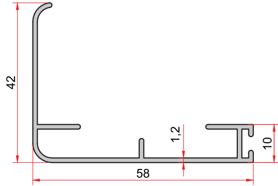
KOD-CODE TEORİK AĞIRLIK 1090 0,449 Kg/m THEORETICAL WEIGHT
