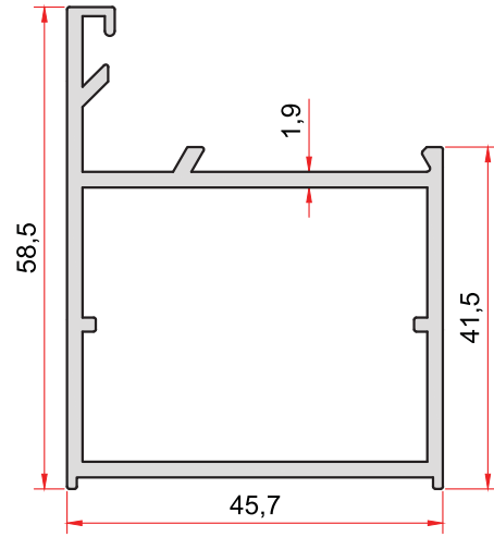
KOD-CODE TEORİK AĞIRLIK THEORETICAL WEIGHT 882 1,010 Kg/m
