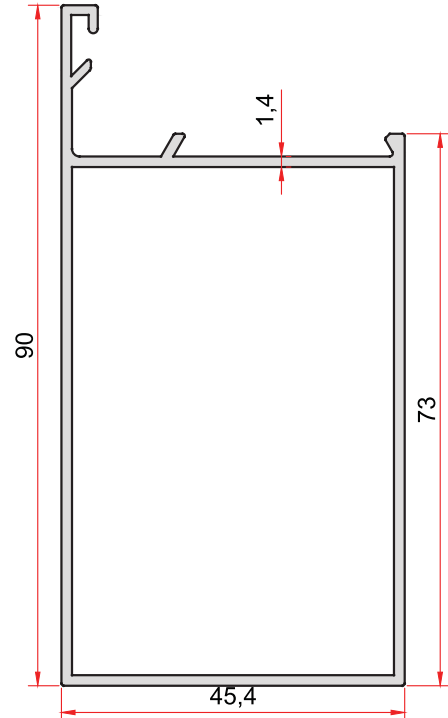
KOD-CODE TEORİK AĞIRLIK 829 THEORETICAL WEIGHT 0,985 Kg/m
