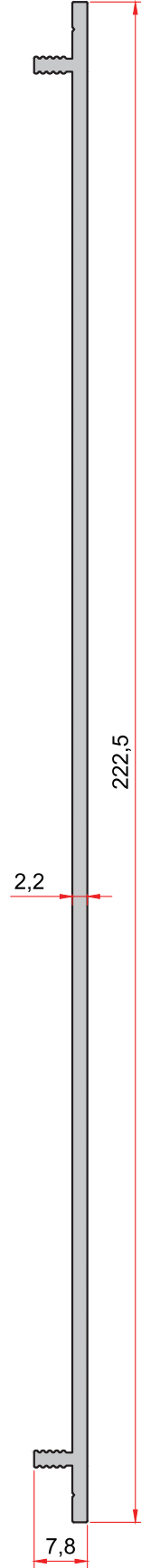
TEORİK AĞIRLIK THEORETICAL WEIGHT KOD-CODE 1094 1,388 Kg/m
