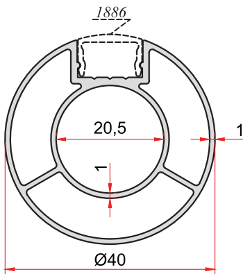
KOD-CODE TEORİK AĞIRLIK 2000 THEORETICAL WEIGHT 0,607 Kg/m
