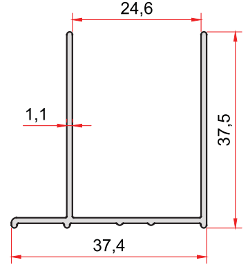
KOD-CODE TEORİK AĞIRLIK THEORETICAL WEIGHT 1774 0,321 Kg/m
