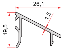
KOD-CODE TEORİK AĞIRLIK 1033 THEORETICAL WEIGHT 0,208 Kg/m
