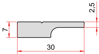
KOD-CODE TEORİK AĞIRLIK THEORETICAL WEIGHT 1476 0,392 Kg/m
