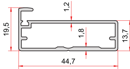
KOD-CODE TEORİK AĞIRLIK 1421 THEORETICAL WEIGHT 0,446 Kg/m
