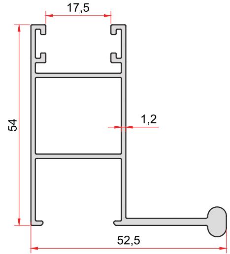
KOD-CODE TEORİK AĞIRLIK 1014 THEORETICAL WEIGHT 0,776 Kg/m
