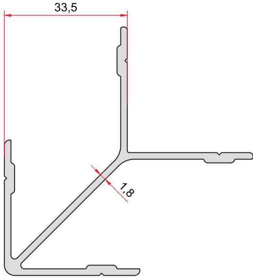
KOD-CODE TEORİK AĞIRLIK THEORETICAL WEIGHT 7027 0,980 Kg/m
