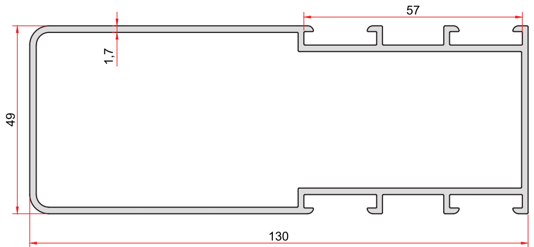
KOD-CODE TEORİK AĞIRLIK THEORETICAL WEIGHT 1188 1,782 Kg/m
