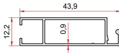
KOD-CODE TEORİK AĞIRLIK THEORETICAL WEIGHT 768 0,283 Kg/m
