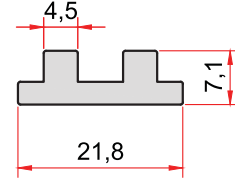
KOD-CODE TEORİK AĞIRLIK THEORETICAL WEIGHT 868 0,275 Kg/m
