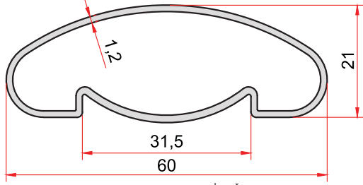
KOD-CODE TEORİK AĞIRLIK THEORETICAL WEIGHT 5033 0,489 Kg/m
