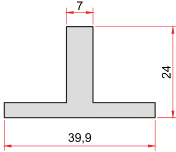
KOD-CODE TEORİK AĞIRLIK 1416 0,805 Kg/m THEORETICAL WEIGHT
