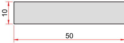
KOD-CODE TEORİK AĞIRLIK THEORETICAL WEIGHT 71 1,350 Kg/m
