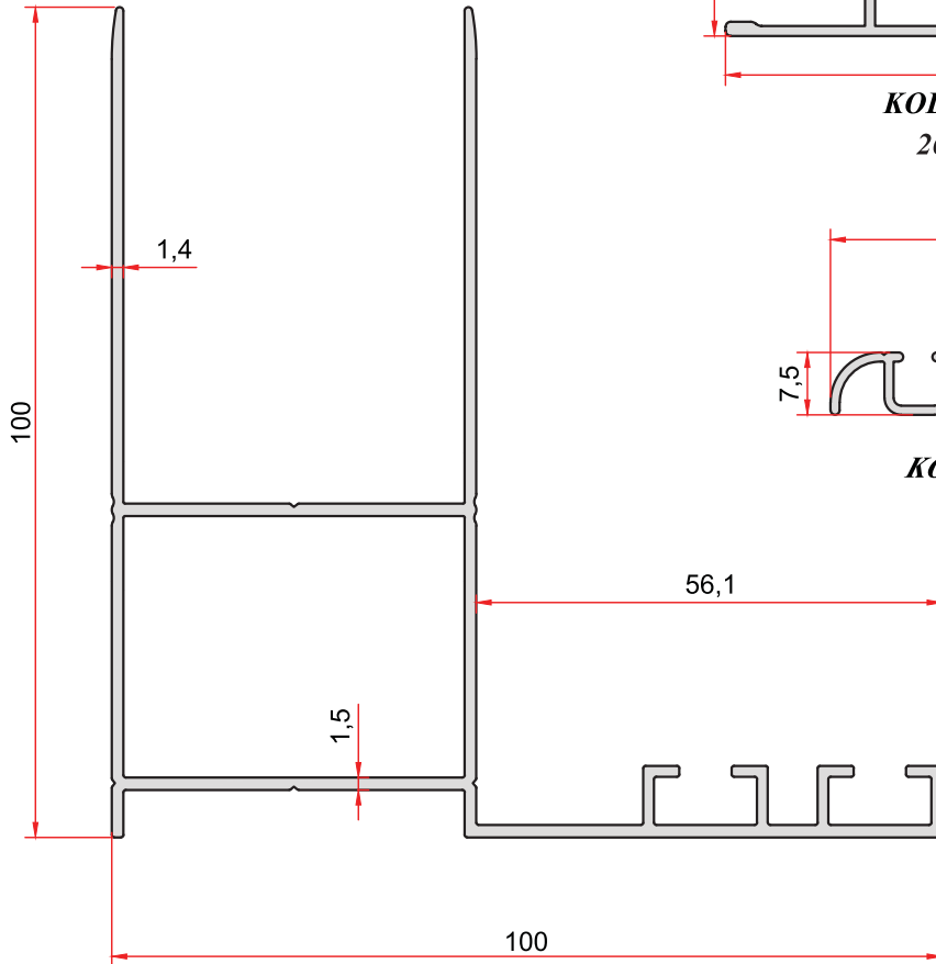
KOD-CODE TEORİK AĞIRLIK THEORETICAL WEIGHT 2736 1,447 Kg/m
