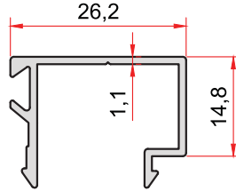
KOD-CODE TEORİK AĞIRLIK 1087 THEORETICAL WEIGHT 0,233 Kg/m
