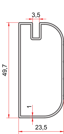
KOD-CODE TEORİK AĞIRLIK 877 THEORETICAL WEIGHT 0,402 Kg/m
