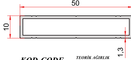
KOD-CODE TEORİK AĞIRLIK THEORETICAL WEIGHT 5088 0,400 Kg/m
