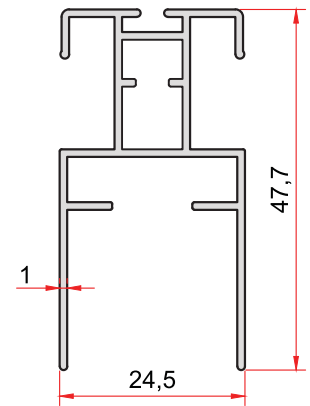
KOD-CODE TEORİK AĞIRLIK THEORETICAL WEIGHT 1306 0,459 Kg/m
