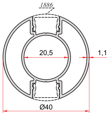
KOD-CODE TEORİK AĞIRLIK 5012 THEORETICAL WEIGHT 0,600 Kg/m
