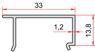
KOD-CODE TEORİK AĞIRLIK 1023 THEORETICAL WEIGHT 0,211 Kg/m
