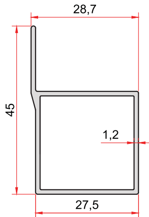
KOD-CODE TEORİK AĞIRLIK THEORETICAL WEIGHT 1017 0,406 Kg/m
