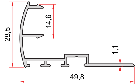
KOD-CODE TEORİK AĞIRLIK THEORETICAL WEIGHT 1137 0,324 Kg/m
