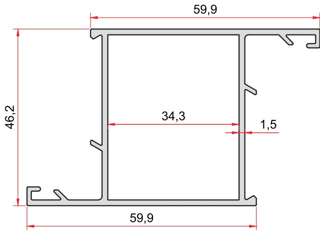
KOD-CODE TEORİK AĞIRLIK THEORETICAL WEIGHT 906 0,921 Kg/m
