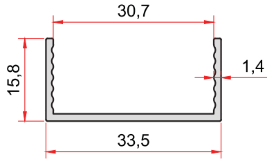
KOD-CODE TEORİK AĞIRLIK 2627 0,224 Kg/m THEORETICAL WEIGHT
