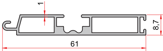
KOD-CODE TEORİK AĞIRLIK 1093 0,437 Kg/m THEORETICAL WEIGHT
