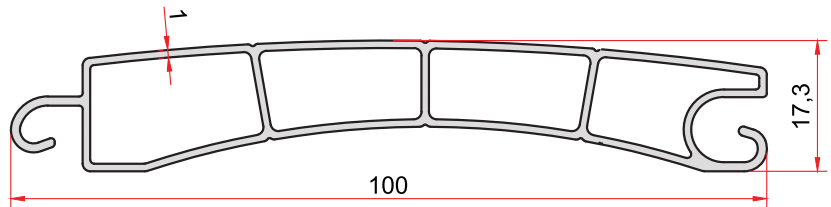
KOD-CODE TEORİK AĞIRLIK THEORETICAL WEIGHT 2311 0,748 Kg/m
