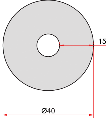
KOD-CODE TEORİK AĞIRLIK THEORETICAL WEIGHT 1853 3,181 Kg/m
