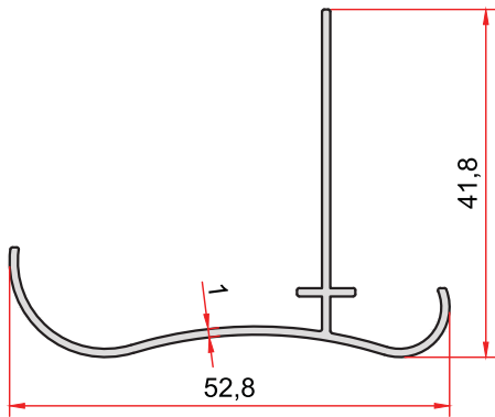
KOD-CODE TEORİK AĞIRLIK THEORETICAL WEIGHT 1242 0,297 Kg/m
