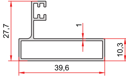
KOD-CODE TEORİK AĞIRLIK 2763 THEORETICAL WEIGHT 0,356 Kg/m
