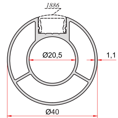
KOD-CODE TEORİK AĞIRLIK 1931 THEORETICAL WEIGHT 0,672 Kg/m
