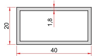
KOD-CODE TEORİK AĞIRLIK 31 THEORETICAL WEIGHT 0,548 Kg/m
