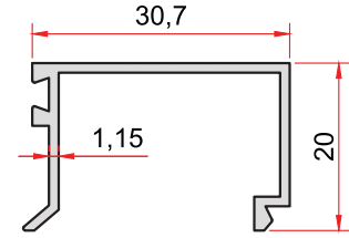
KOD-CODE TEORİK AĞIRLIK THEORETICAL WEIGHT 859 0,248 Kg/m
