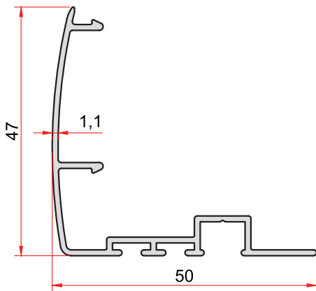
KOD-CODE TEORİK AĞIRLIK THEORETICAL WEIGHT SS-602-11 0,402 Kg/m
