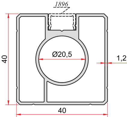
KOD-CODE TEORİK AĞIRLIK 1975 THEORETICAL WEIGHT 0,845 Kg/m
