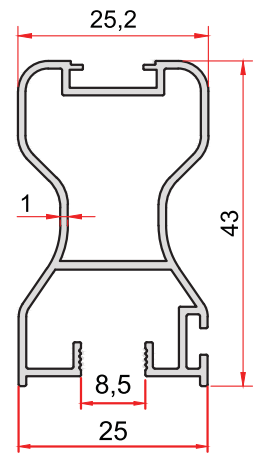
KOD-CODE TEORİK AĞIRLIK THEORETICAL WEIGHT 1459 0,451 Kg/m
