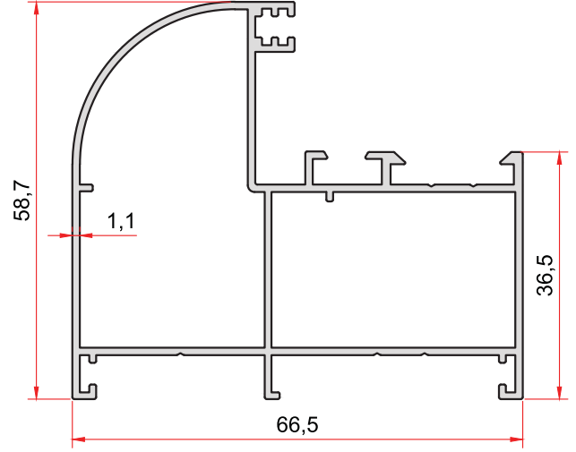
KOD-CODE TEORİK AĞIRLIK THEORETICAL WEIGHT 1129 0,937 Kg/m
