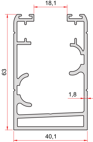
KOD-CODE TEORİK AĞIRLIK THEORETICAL WEIGHT 2371 1,328 Kg/m
