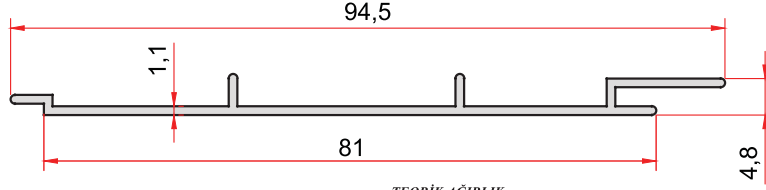
KOD-CODE TEORİK AĞIRLIK THEORETICAL WEIGHT 834 0,351 Kg/m
