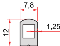
KOD-CODE TEORİK AĞIRLIK THEORETICAL WEIGHT 1494 0,156 Kg/m
