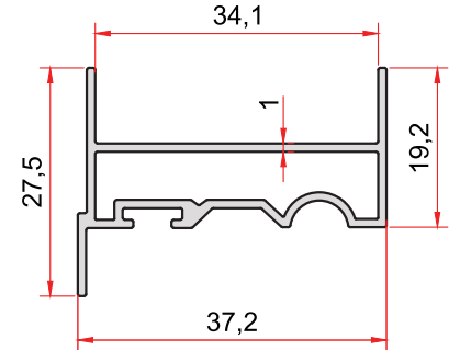
KOD-CODE TEORİK AĞIRLIK 2299 0,354 Kg/m THEORETICAL WEIGHT
