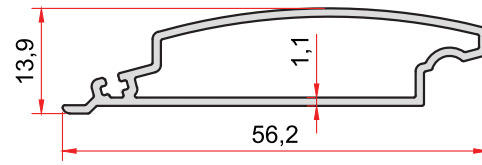
KOD-CODE TEORİK AĞIRLIK 1015 0,365 Kg/m THEORETICAL WEIGHT
