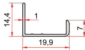
KOD-CODE 778 TEORİK AĞIRLIK 0,103 Kg/m THEORETICAL WEIGHT
