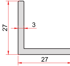
KOD-CODE TEORİK AĞIRLIK THEORETICAL WEIGHT 775 0,413 Kg/m
