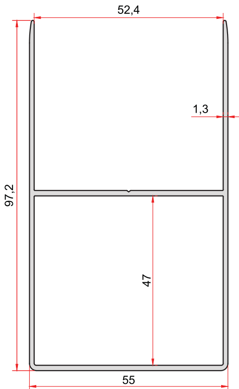
KOD-CODE TEORİK AĞIRLIK THEORETICAL WEIGHT 2630 1,096 Kg/m
