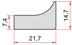
KOD-CODE TEORİK AĞIRLIK THEORETICAL WEIGHT 1497 0,505 Kg/m
