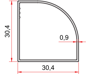
KOD-CODE 774 TEORİK AĞIRLIK 0,267 Kg/m THEORETICAL WEIGHT
