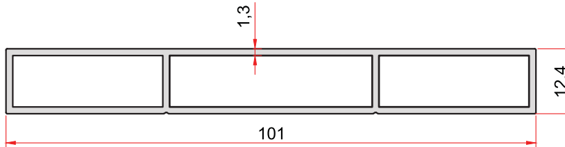
KOD-CODE TEORİK AĞIRLIK THEORETICAL WEIGHT 2442 0,845 Kg/m
