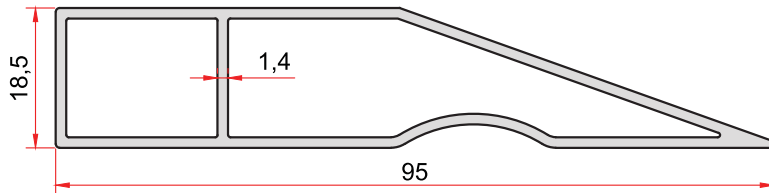
KOD-CODE TEORİK AĞIRLIK 4000 THEORETICAL WEIGHT 0,837 Kg/m
