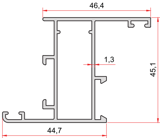
KOD-CODE TEORİK AĞIRLIK THEORETICAL WEIGHT 1077 0,788 Kg/m
