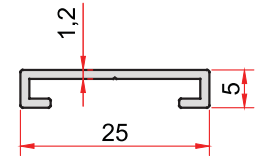
KOD-CODE TEORİK AĞIRLIK 837 THEORETICAL WEIGHT 0,124 Kg/m
