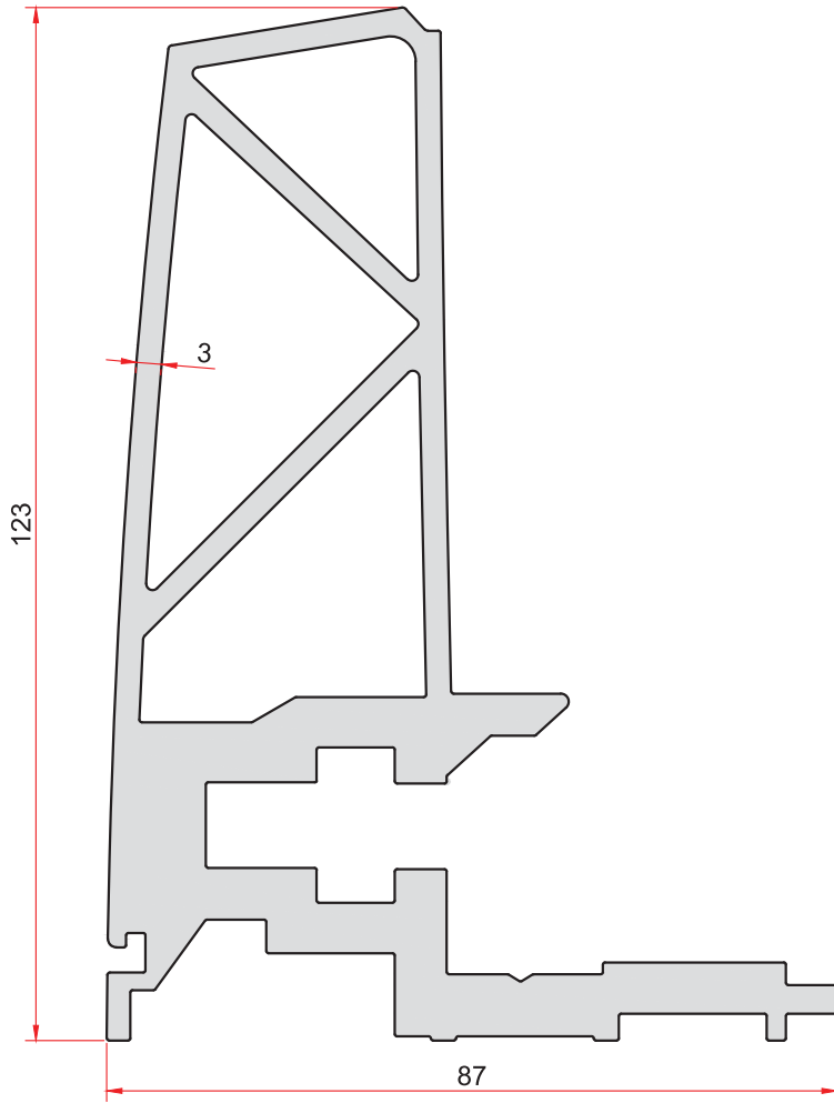
KOD-CODE TEORİK AĞIRLIK THEORETICAL WEIGHT 1995 5,581 Kg/m
