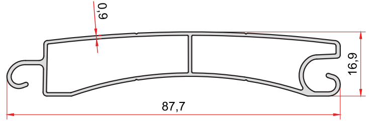
KOD-CODE TEORİK AĞIRLIK THEORETICAL WEIGHT 2301 0,572 Kg/m
