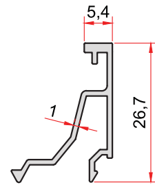
KOD-CODE TEORİK AĞIRLIK 1133 THEORETICAL WEIGHT 0,189 Kg/m
