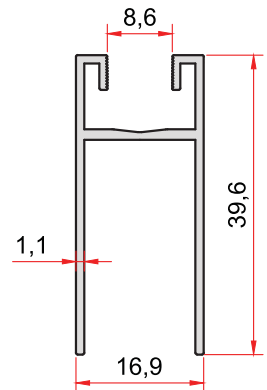
KOD-CODE TEORİK AĞIRLIK THEORETICAL WEIGHT 1400 0,324 Kg/m
