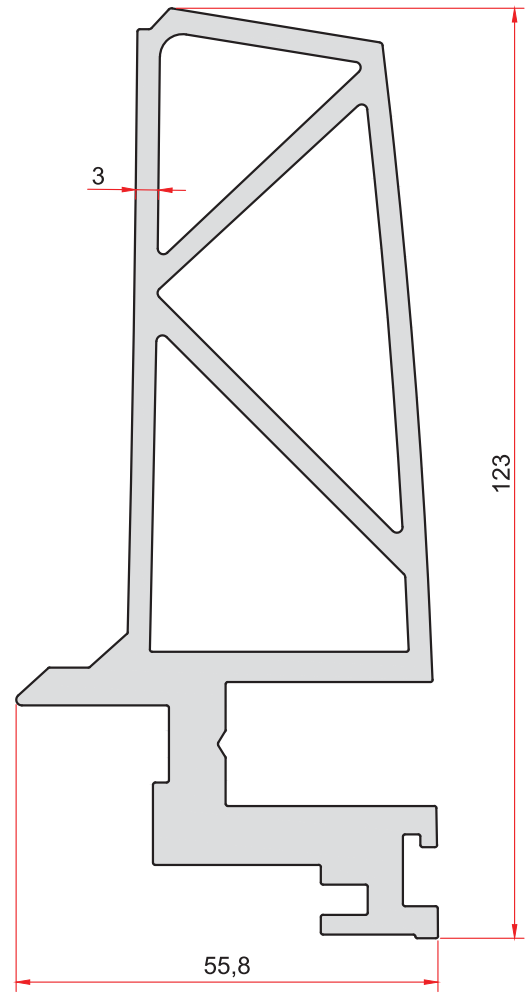
KOD-CODE TEORİK AĞIRLIK THEORETICAL WEIGHT 1994 4,282 Kg/m
