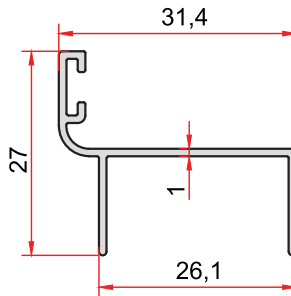
KOD-CODE 2757 TEORİK AĞIRLIK 0,208 THEORETICAL WEIGHT Kg/m
