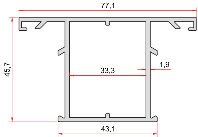
KOD-CODE TEORİK AĞIRLIK THEORETICAL WEIGHT 880 1,177 Kg/m
