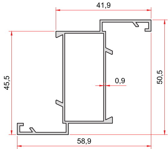
KOD-CODE TEORİK AĞIRLIK THEORETICAL WEIGHT 861 0,537 Kg/m
