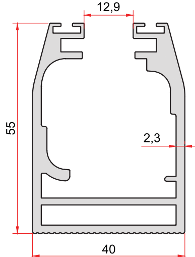
KOD-CODE TEORİK AĞIRLIK 2255 THEORETICAL WEIGHT 1,477 Kg/m
