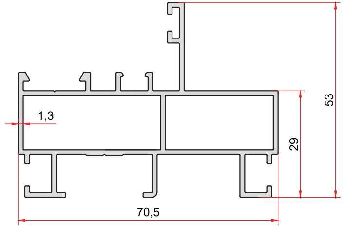
KOD-CODE TEORİK AĞIRLIK THEORETICAL WEIGHT 7034 1,085 Kg/m
