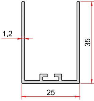
KOD-CODE TEORİK AĞIRLIK THEORETICAL WEIGHT 2437 0,332 Kg/m
