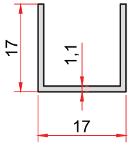
KOD-CODE TEORİK AĞIRLIK THEORETICAL WEIGHT 83 0,146 Kg/m
