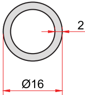
KOD-CODE 1943 TEORİK AĞIRLIK THEORETICAL WEIGHT 0,238 Kg/m
