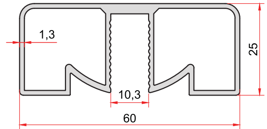
KOD-CODE TEORİK AĞIRLIK THEORETICAL WEIGHT 1903 0,804 Kg/m
