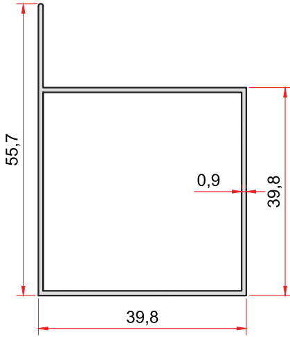
KOD-CODE TEORİK AĞIRLIK THEORETICAL WEIGHT 1435 0,416 Kg/m
