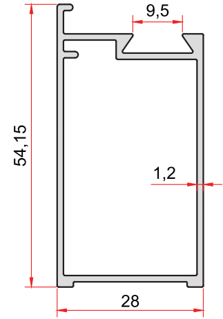
KOD-CODE TEORİK AĞIRLIK THEORETICAL WEIGHT 1032 0,575 Kg/m
