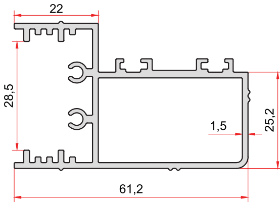
KOD-CODE TEORİK AĞIRLIK 2631 THEORETICAL WEIGHT 0,726 Kg/m
