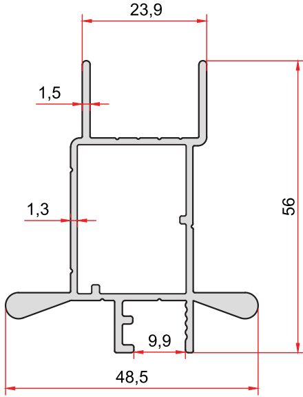
KOD-CODE TEORİK AĞIRLIK THEORETICAL WEIGHT 2724 0,829 Kg/m
