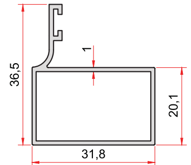
KOD-CODE TEORİK AĞIRLIK 2262 0,359 Kg/m THEORETICAL WEIGHT
