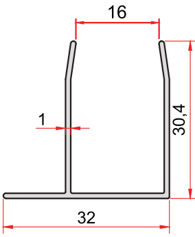
KOD-CODE TEORİK AĞIRLIK THEORETICAL WEIGHT 1767 0,243 Kg/m
