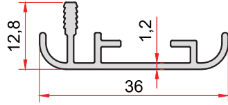
KOD-CODE TEORİK AĞIRLIK 1030 0,254 Kg/m THEORETICAL WEIGHT
