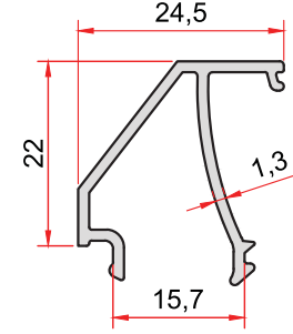
KOD-CODE TEORİK AĞIRLIK THEORETICAL WEIGHT 1979 0,267 Kg/m
