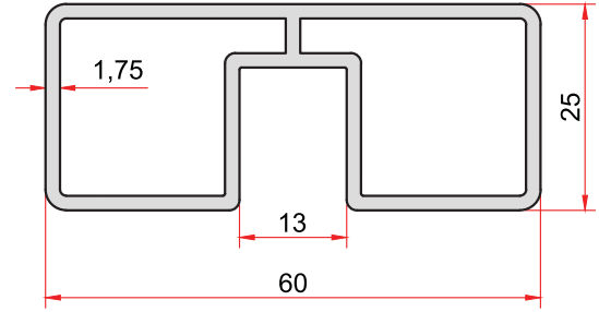
KOD-CODE TEORİK AĞIRLIK THEORETICAL WEIGHT 1997 0,937 Kg/m
