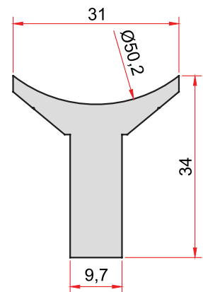
KOD-CODE TEORİK AĞIRLIK 1862 1,007 Kg/m THEORETICAL WEIGHT
