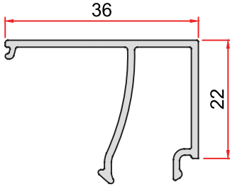
KOD-CODE TEORİK AĞIRLIK THEORETICAL WEIGHT CC-1360-13 0,327 Kg/m
