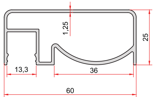
KOD-CODE TEORİK AĞIRLIK THEORETICAL WEIGHT 1961 0,675 Kg/m
