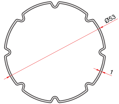
KOD-CODE TEORİK AĞIRLIK THEORETICAL WEIGHT 1445 0,478 Kg/m
