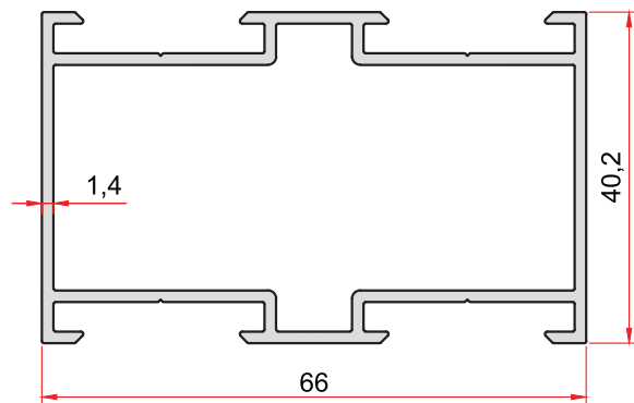
KOD-CODE TEORİK AĞIRLIK THEORETICAL WEIGHT 1036 0,944 Kg/m
