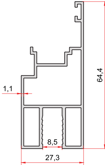
KOD-CODE TEORİK AĞIRLIK 7042 THEORETICAL WEIGHT 0,696 Kg/m
