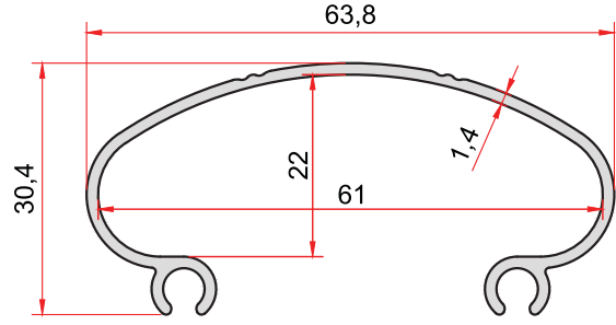
KOD-CODE TEORİK AĞIRLIK THEORETICAL WEIGHT 5066 0,505 Kg/m
