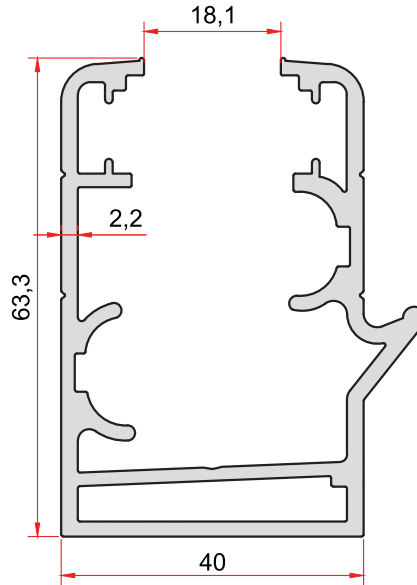
KOD-CODE TEORİK AĞIRLIK THEORETICAL WEIGHT 2272 1,545 Kg/m
