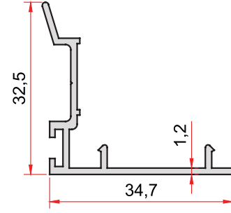
KOD-CODE TEORİK AĞIRLIK 819 THEORETICAL WEIGHT 0,283 Kg/m
