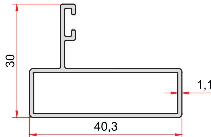
KOD-CODE TEORİK AĞIRLIK 2256 0,378 Kg/m THEORETICAL WEIGHT
