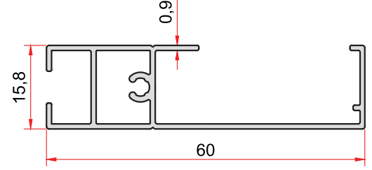
KOD-CODE TEORİK AĞIRLIK THEORETICAL WEIGHT 1765 0,391 Kg/m
