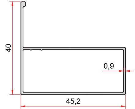
KOD-CODE 771 TEORİK AĞIRLIK 0,364 Kg/m THEORETICAL WEIGHT
