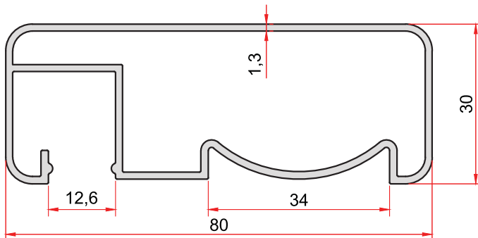
KOD-CODE TEORİK AĞIRLIK 5007 THEORETICAL WEIGHT 0,915 Kg/m
