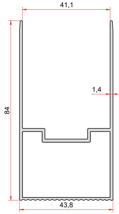
KOD-CODE TEORİK AĞIRLIK THEORETICAL WEIGHT 2274 0,929 Kg/m
