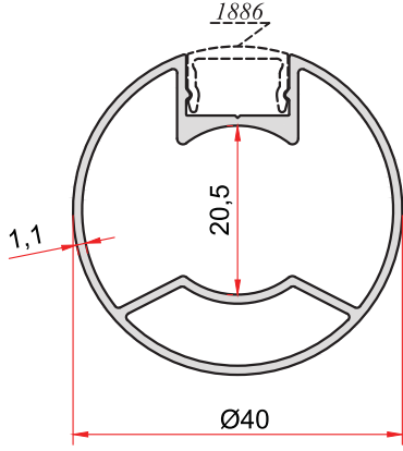
KOD-CODE TEORİK AĞIRLIK THEORETICAL WEIGHT 5072 0,543 Kg/m
