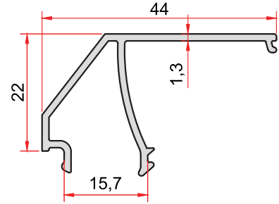
KOD-CODE TEORİK AĞIRLIK THEORETICAL WEIGHT 1981 0,335 Kg/m
