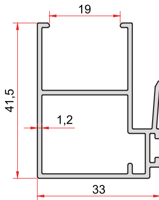
KOD-CODE TEORİK AĞIRLIK 1003 THEORETICAL WEIGHT 0,540 Kg/m
