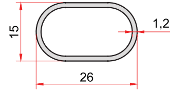
KOD-CODE TEORİK AĞIRLIK THEORETICAL WEIGHT 802 0,219 Kg/m
