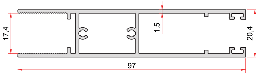
KOD-CODE TEORİK AĞIRLIK 2380 THEORETICAL WEIGHT 1,036 Kg/m
