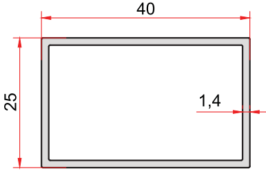
KOD-CODE TEORİK AĞIRLIK THEORETICAL WEIGHT 5078 0,470 Kg/m
