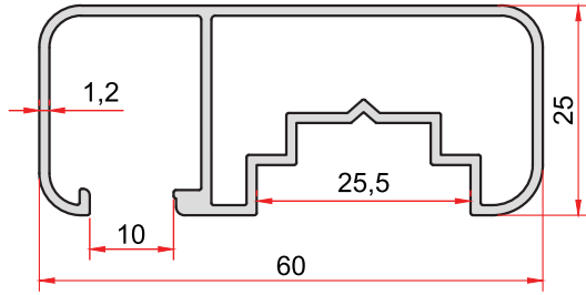
KOD-CODE TEORİK AĞIRLIK 5042 THEORETICAL WEIGHT 0,645 Kg/m
