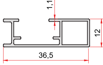
KOD-CODE TEORİK AĞIRLIK THEORETICAL WEIGHT 1761 0,259 Kg/m
