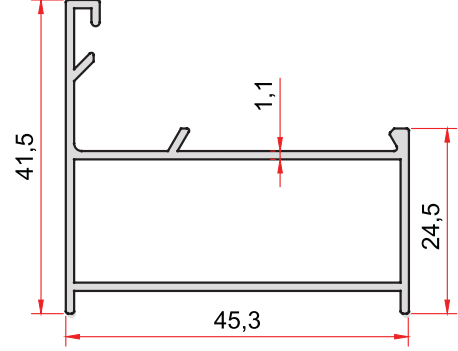
KOD-CODE TEORİK AĞIRLIK THEORETICAL WEIGHT 823 0,499 Kg/m
