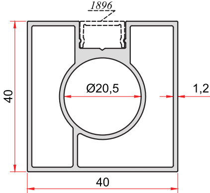
KOD-CODE TEORİK AĞIRLIK 1895 THEORETICAL WEIGHT 0,845 Kg/m
