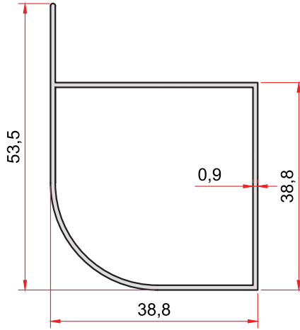
KOD-CODE TEORİK AĞIRLIK THEORETICAL WEIGHT 1436 0,383 Kg/m
