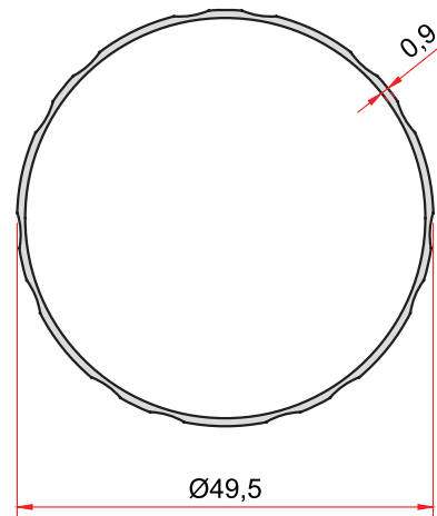
KOD-CODE TEORİK AĞIRLIK THEORETICAL WEIGHT 4021 0,356 Kg/m
