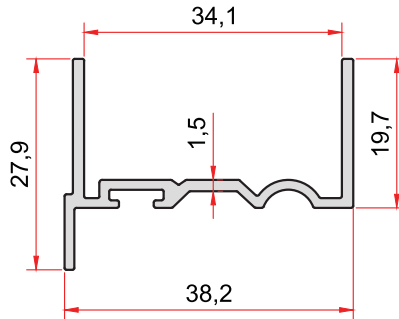
KOD-CODE TEORİK AĞIRLIK 2626 0,356 Kg/m THEORETICAL WEIGHT
