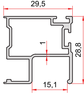
KOD-CODE TEORİK AĞIRLIK 1465 THEORETICAL WEIGHT 0,405 Kg/m
