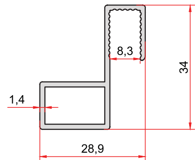
KOD-CODE TEORİK AĞIRLIK 2682 THEORETICAL WEIGHT 0,375 Kg/m
