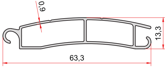
KOD-CODE TEORİK AĞIRLIK THEORETICAL WEIGHT 2313 0,402 Kg/m
