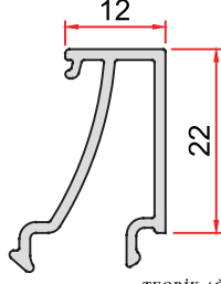
KOD-CODE TEORİK AĞIRLIK THEORETICAL WEIGHT CC-1120-13 0,254 Kg/m
