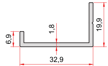
KOD-CODE TEORİK AĞIRLIK 1446 0,273 Kg/m THEORETICAL WEIGHT
