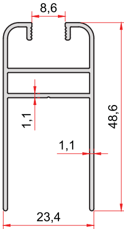
KOD-CODE TEORİK AĞIRLIK THEORETICAL WEIGHT 1360 0,464 Kg/m
