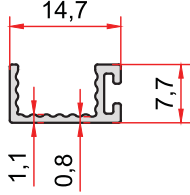
KOD-CODE 2720 TEORİK AĞIRLIK 0,092 THEORETICAL WEIGHT Kg/m
