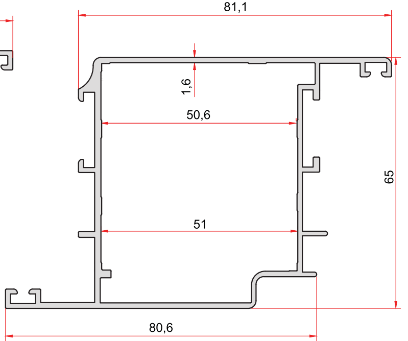
KOD-CODE TEORİK AĞIRLIK THEORETICAL WEIGHT 7038 1,417 Kg/m
