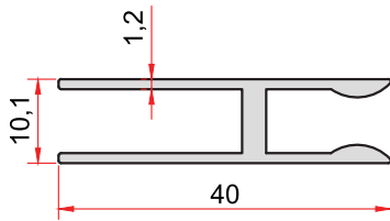
KOD-CODE TEORİK AĞIRLIK THEORETICAL WEIGHT 869 0,340 Kg/m
