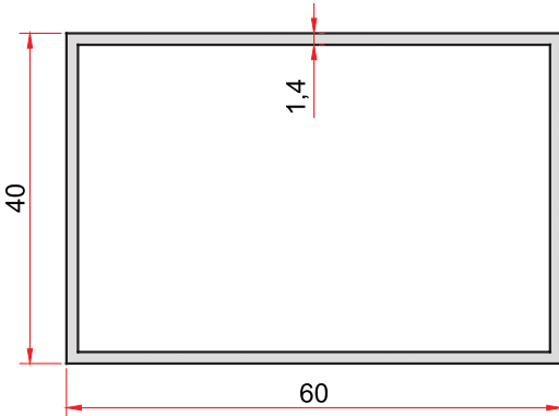
KOD-CODE TEORİK AĞIRLIK THEORETICAL WEIGHT 24 0,734 Kg/m
