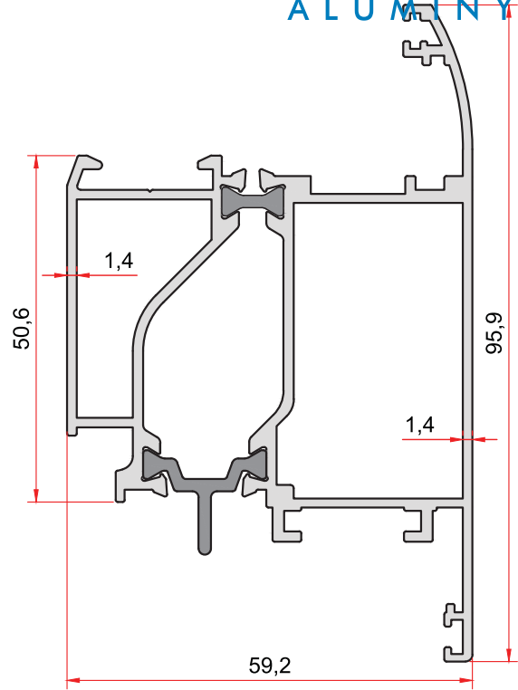
KOD-CODE TEORİK AĞIRLIK İD-601-15 THEORETICAL WEIGHT 1,763 Kg/m
