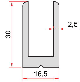
KOD-CODE TEORİK AĞIRLIK 841 THEORETICAL WEIGHT 0,553 Kg/m
