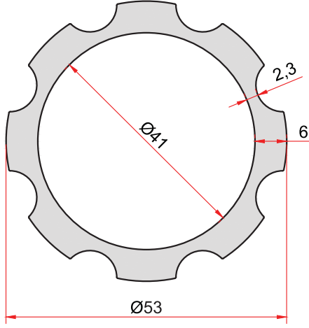
KOD-CODE TEORİK AĞIRLIK THEORETICAL WEIGHT 1909 1,845 Kg/m
