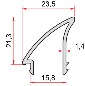
KOD-CODE TEORİK AĞIRLIK THEORETICAL WEIGHT 5019 0,251 Kg/m
