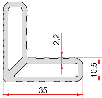
KOD-CODE TEORİK AĞIRLIK KT-1105-00 THEORETICAL WEIGHT 0,793 Kg/m
