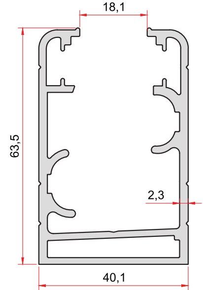
KOD-CODE TEORİK AĞIRLIK THEORETICAL WEIGHT 2393 1,477 Kg/m
