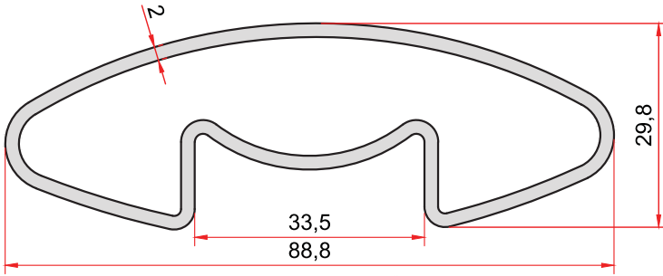
KOD-CODE TEORİK AĞIRLIK THEORETICAL WEIGHT 1928 1,188 Kg/m
