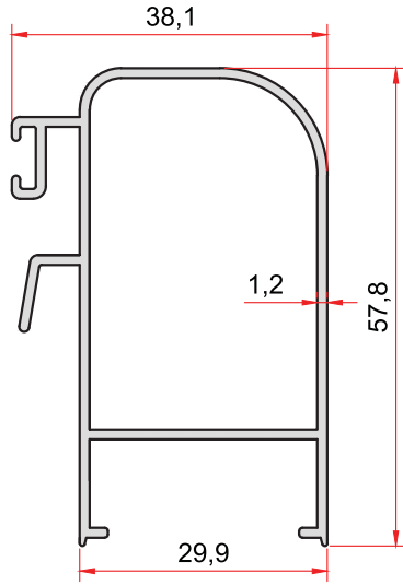
KOD-CODE TEORİK AĞIRLIK THEORETICAL WEIGHT 874 0,656 Kg/m
