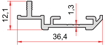
KOD-CODE TEORİK AĞIRLIK 1107 0,238 Kg/m THEORETICAL WEIGHT
