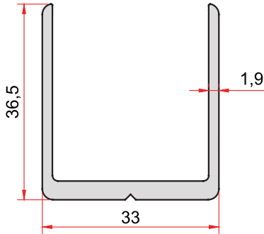
KOD-CODE TEORİK AĞIRLIK 842 THEORETICAL WEIGHT 0,640 Kg/m
