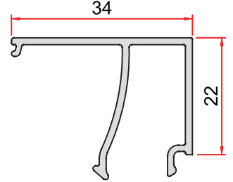
KOD-CODE TEORİK AĞIRLIK THEORETICAL WEIGHT CC-1340-13 0,320 Kg/m
