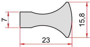
KOD-CODE TEORİK AĞIRLIK THEORETICAL WEIGHT 1439 0,489 Kg/m
