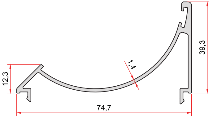
KOD-CODE TEORİK AĞIRLIK 1202 THEORETICAL WEIGHT 0,621 Kg/m
