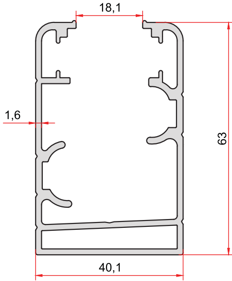
KOD-CODE TEORİK AĞIRLIK 2680 THEORETICAL WEIGHT 1,231 Kg/m
