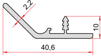
KOD-CODE TEORİK AĞIRLIK THEORETICAL WEIGHT 1474 0,324 Kg/m
