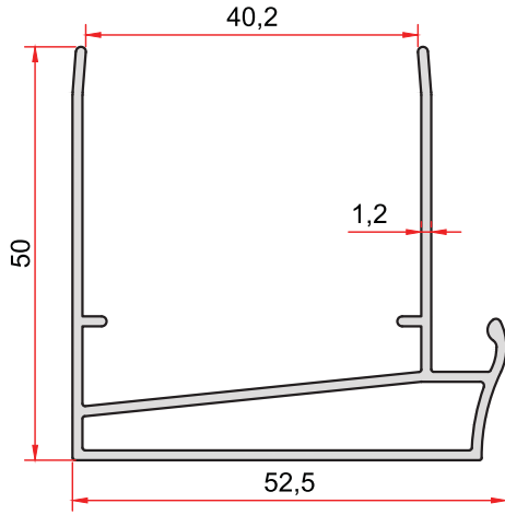
KOD-CODE TEORİK AĞIRLIK THEORETICAL WEIGHT 2664 0,680 Kg/m
