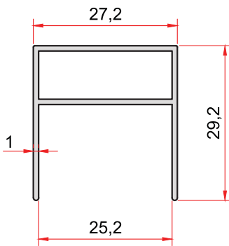
KOD-CODE TEORİK AĞIRLIK THEORETICAL WEIGHT 1304 0,294 Kg/m
