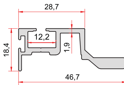
KOD-CODE TEORİK AĞIRLIK 1467 0,581 Kg/m THEORETICAL WEIGHT
