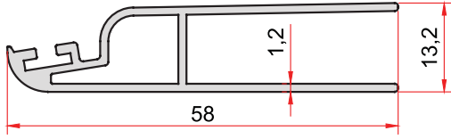
KOD-CODE TEORİK AĞIRLIK THEORETICAL WEIGHT 798 0,465 Kg/m
