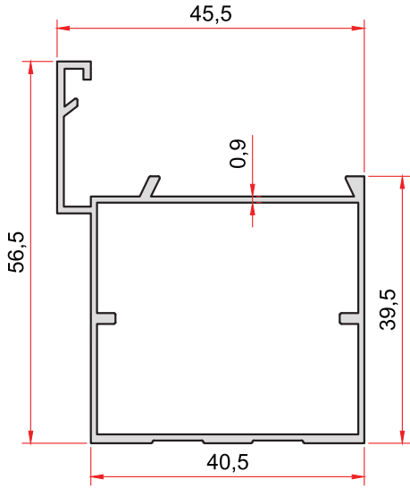
KOD-CODE 858 TEORİK AĞIRLIK THEORETICAL WEIGHT 0,543 Kg/m
