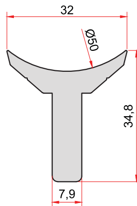
KOD-CODE TEORİK AĞIRLIK 1892 0,934 Kg/m THEORETICAL WEIGHT
