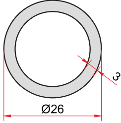
KOD-CODE TEORİK AĞIRLIK 5084 THEORETICAL WEIGHT 0,583 Kg/m
