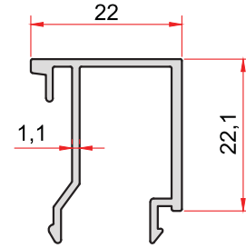
KOD-CODE TEORİK AĞIRLIK 1120 THEORETICAL WEIGHT 0,278 Kg/m
