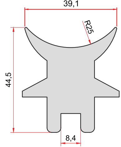
KOD-CODE TEORİK AĞIRLIK 1966 2,397 Kg/m THEORETICAL WEIGHT
