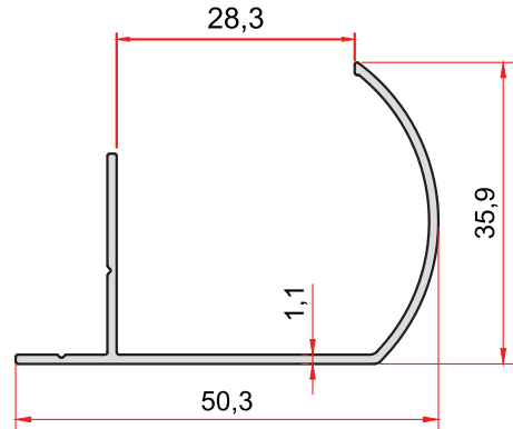
KOD-CODE TEORİK AĞIRLIK THEORETICAL WEIGHT 1756 0,313 Kg/m
