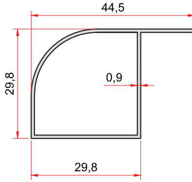
KOD-CODE TEORİK AĞIRLIK THEORETICAL WEIGHT 1434 0,297 Kg/m
