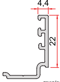
KOD-CODE TEORİK AĞIRLIK THEORETICAL WEIGHT CC-1044-15 0,212 Kg/m
