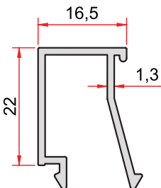
KOD-CODE TEORİK AĞIRLIK THEORETICAL WEIGHT 847 0,262 Kg/m
