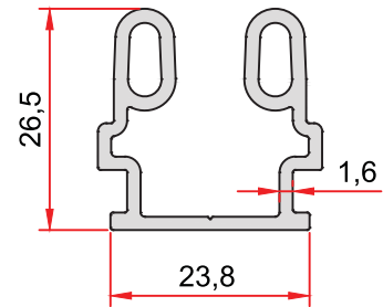
KOD-CODE TEORİK AĞIRLIK AO-1051-16 THEORETICAL WEIGHT 0,522 Kg/m
