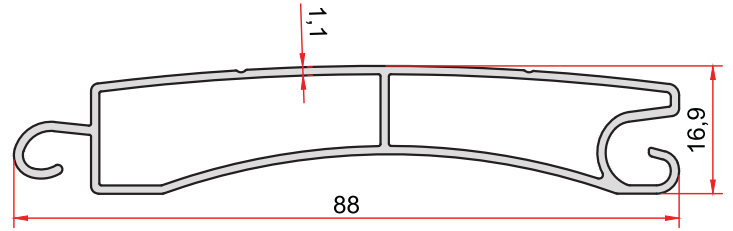
KOD-CODE TEORİK AĞIRLIK THEORETICAL WEIGHT 2315 0,667 Kg/m
