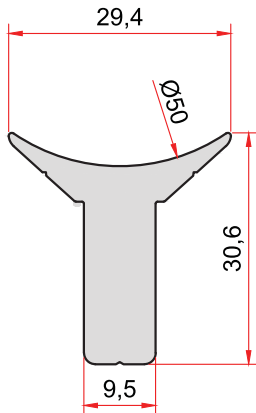
KOD-CODE TEORİK AĞIRLIK 1942 0,853 Kg/m THEORETICAL WEIGHT
