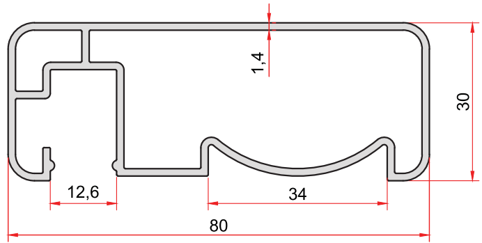
KOD-CODE TEORİK AĞIRLIK 1944 THEORETICAL WEIGHT 1,004 Kg/m
