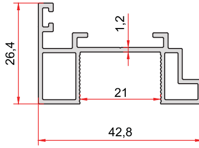
KOD-CODE TEORİK AĞIRLIK 2733 THEORETICAL WEIGHT 0,443 Kg/m
