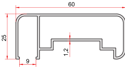
KOD-CODE TEORİK AĞIRLIK 5079 THEORETICAL WEIGHT 0,607 Kg/m
