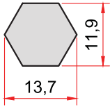
KOD-CODE 2273 TEORİK AĞIRLIK 0,332 THEORETICAL WEIGHT Kg/m
