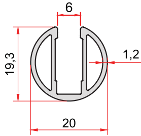
KOD-CODE TEORİK AĞIRLIK THEORETICAL WEIGHT 1769 0,275 Kg/m
