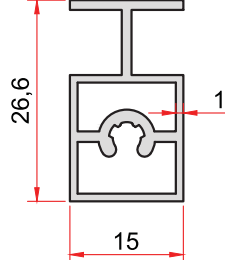
KOD-CODE TEORİK AĞIRLIK THEORETICAL WEIGHT 1369 0,327 Kg/m
