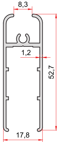
KOD-CODE TEORİK AĞIRLIK THEORETICAL WEIGHT 1396 0,486 Kg/m
