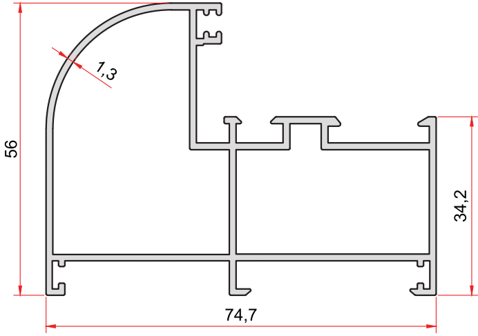
KOD-CODE TEORİK AĞIRLIK THEORETICAL WEIGHT 1119 1,129 Kg/m
