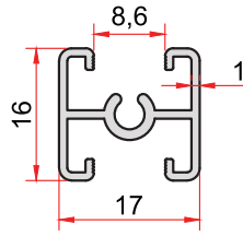
KOD-CODE TEORİK AĞIRLIK THEORETICAL WEIGHT 1398 0,200 Kg/m
