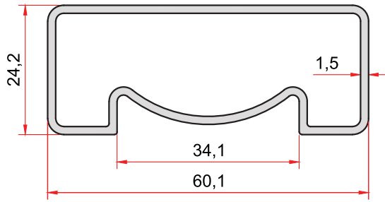
KOD-CODE TEORİK AĞIRLIK 1874 THEORETICAL WEIGHT 0,707 Kg/m
