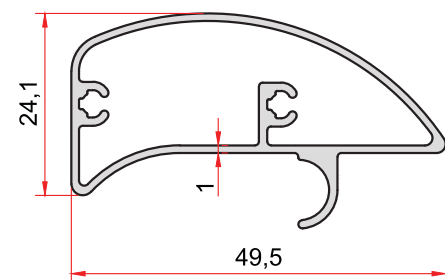
KOD-CODE TEORİK AĞIRLIK 1770 THEORETICAL WEIGHT 0,475 Kg/m
