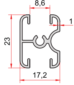
KOD-CODE TEORİK AĞIRLIK THEORETICAL WEIGHT 1394 0,243 Kg/m
