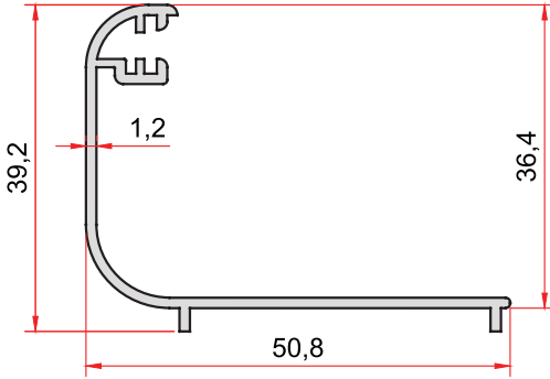
KOD-CODE TEORİK AĞIRLIK THEORETICAL WEIGHT 800 0,370 Kg/m
