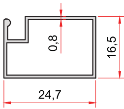
KOD-CODE TEORİK AĞIRLIK THEORETICAL WEIGHT 1301 0,189 Kg/m
