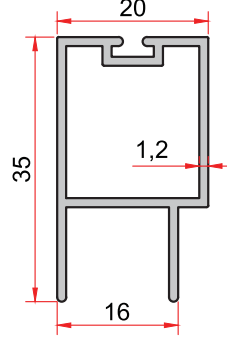
KOD-CODE TEORİK AĞIRLIK THEORETICAL WEIGHT 1092 0,365 Kg/m
