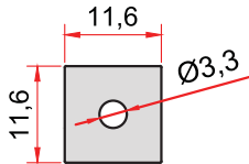
KOD-CODE TEORİK AĞIRLIK THEORETICAL WEIGHT 1499 0,797 Kg/m
