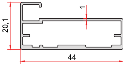
KOD-CODE TEORİK AĞIRLIK 1460 THEORETICAL WEIGHT 0,410 Kg/m
