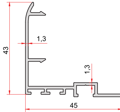
KOD-CODE TEORİK AĞIRLIK SS-401-13 THEORETICAL WEIGHT 0,432 Kg/m
