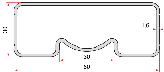
KOD-CODE TEORİK AĞIRLIK 1976 THEORETICAL WEIGHT 0,995 Kg/m
