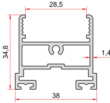
KOD-CODE TEORİK AĞIRLIK 2634 THEORETICAL WEIGHT 0,726 Kg/m
