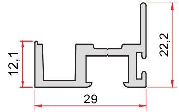
KOD-CODE TEORİK AĞIRLIK 1367 0,408 Kg/m THEORETICAL WEIGHT
