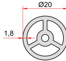
KOD-CODE TEORİK AĞIRLIK THEORETICAL WEIGHT 1496 0,440 Kg/m
