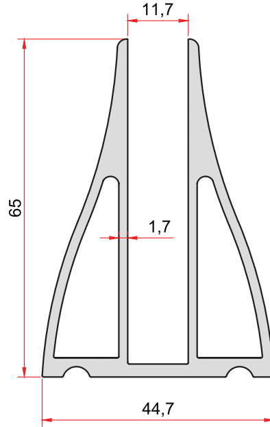
KOD-CODE TEORİK AĞIRLIK THEORETICAL WEIGHT 1953 1,571 Kg/m
