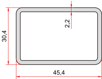
KOD-CODE TEORİK AĞIRLIK THEORETICAL WEIGHT 5055 0,823 Kg/m
