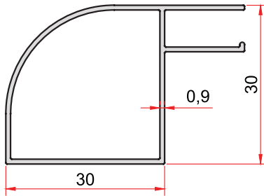
KOD-CODE 772 TEORİK AĞIRLIK 0,337 Kg/m THEORETICAL WEIGHT
