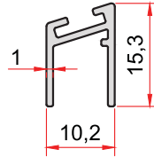
KOD-CODE 2391 TEORİK AĞIRLIK 0,116 THEORETICAL WEIGHT Kg/m
