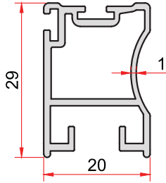
KOD-CODE TEORİK AĞIRLIK THEORETICAL WEIGHT 1397 0,394 Kg/m
