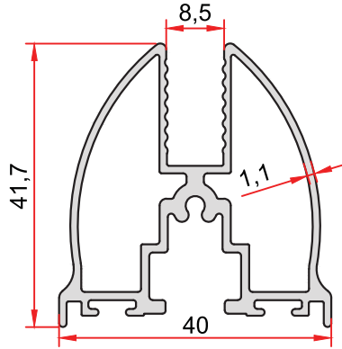
KOD-CODE TEORİK AĞIRLIK 2620 THEORETICAL WEIGHT 0,753 Kg/m
