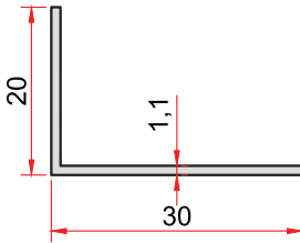
KOD-CODE TEORİK AĞIRLIK THEORETICAL WEIGHT 44 0,145 Kg/m
