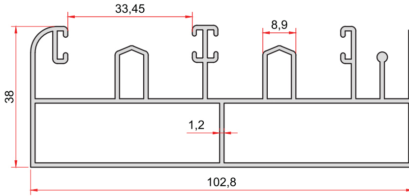
KOD-CODE 873 TEORİK AĞIRLIK THEORETICAL WEIGHT 1,471 Kg/m
