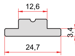
KOD-CODE TEORİK AĞIRLIK THEORETICAL WEIGHT 1440 0,356 Kg/m
