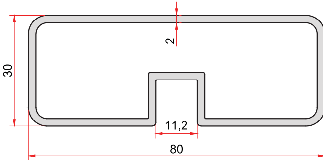
KOD-CODE TEORİK AĞIRLIK THEORETICAL WEIGHT 1954 1,242 Kg/m
