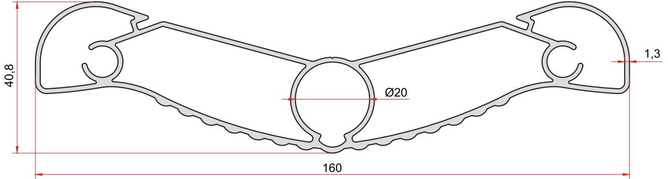
KOD-CODE TEORİK AĞIRLIK 4013 THEORETICAL WEIGHT 1,852 Kg/m
