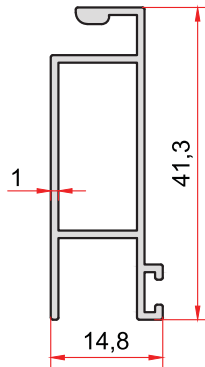
KOD-CODE 7010 TEORİK AĞIRLIK THEORETICAL WEIGHT 0,313 Kg/m
