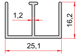
KOD-CODE TEORİK AĞIRLIK THEORETICAL WEIGHT 870 0,235 Kg/m
