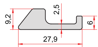
KOD-CODE TEORİK AĞIRLIK THEORETICAL WEIGHT 1490 0,362 Kg/m
