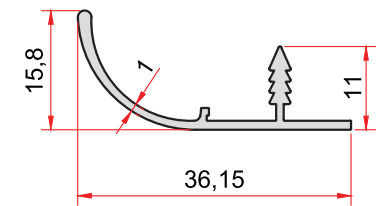
KOD-CODE TEORİK AĞIRLIK THEORETICAL WEIGHT 1484 0,211 Kg/m
