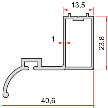
KOD-CODE TEORİK AĞIRLIK 1780 THEORETICAL WEIGHT 0,399 Kg/m
