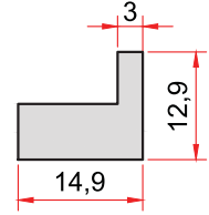
KOD-CODE TEORİK AĞIRLIK THEORETICAL WEIGHT 1409 0,319 Kg/m
