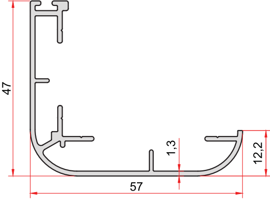
KOD-CODE TEORİK AĞIRLIK 1019 0,588 Kg/m THEORETICAL WEIGHT
