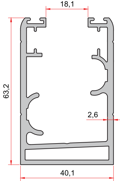
KOD-CODE TEORİK AĞIRLIK THEORETICAL WEIGHT 2448 1,563 Kg/m
