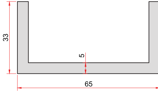
KOD-CODE TEORİK AĞIRLIK THEORETICAL WEIGHT 86 1,633 Kg/m
