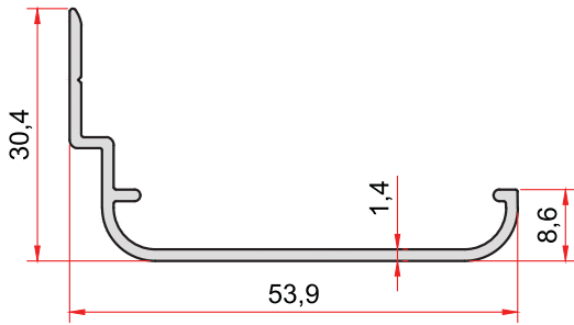
KOD-CODE TEORİK AĞIRLIK THEORETICAL WEIGHT SS-403-14 0,335 Kg/m
