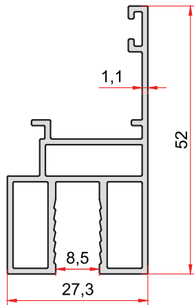
KOD-CODE TEORİK AĞIRLIK 7043 THEORETICAL WEIGHT 0,583 Kg/m
