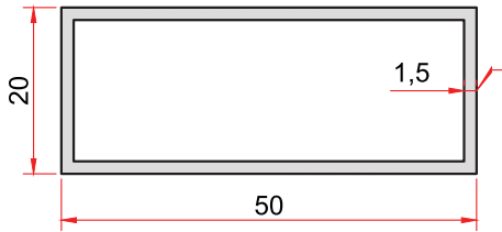
KOD-CODE TEORİK AĞIRLIK THEORETICAL WEIGHT 115 0,542 Kg/m
