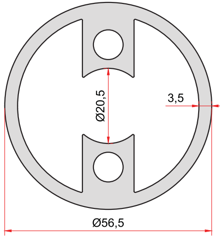
KOD-CODE TEORİK AĞIRLIK 1971 THEORETICAL WEIGHT 2,440 Kg/m
