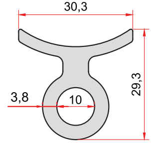
KOD-CODE TEORİK AĞIRLIK THEORETICAL WEIGHT 5032 0,788 Kg/m
