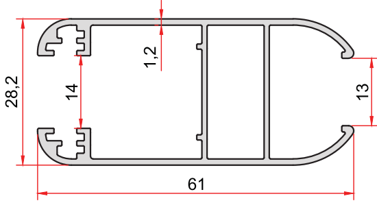
KOD-CODE TEORİK AĞIRLIK THEORETICAL WEIGHT 784 0,685 Kg/m
