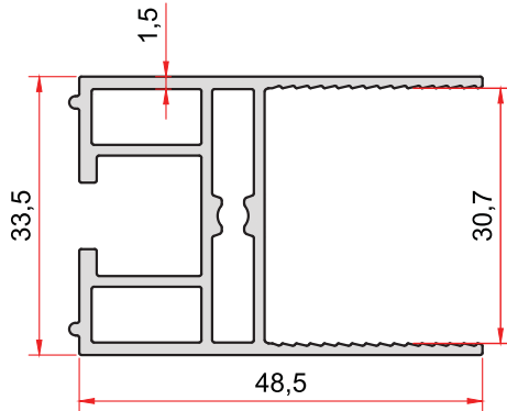
KOD-CODE TEORİK AĞIRLIK THEORETICAL WEIGHT 2370 0,802 Kg/m
