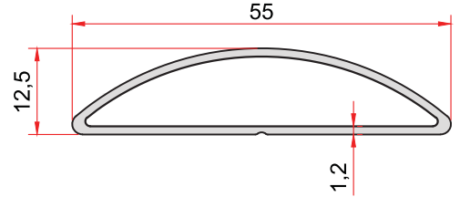
KOD-CODE TEORİK AĞIRLIK THEORETICAL WEIGHT 5069 0,372 Kg/m
