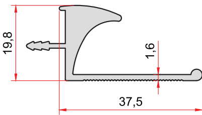
KOD-CODE TEORİK AĞIRLIK THEORETICAL WEIGHT 1383 0,500 Kg/m
