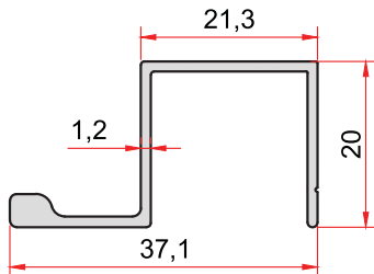
KOD-CODE TEORİK AĞIRLIK 1374 0,281 Kg/m THEORETICAL WEIGHT
