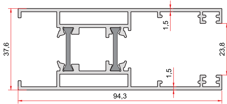
KOD-CODE TEORİK AĞIRLIK MD-101-15 THEORETICAL WEIGHT 1,616 Kg/m
