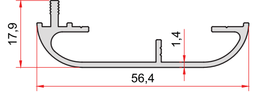
KOD-CODE TEORİK AĞIRLIK 1106 0,421 Kg/m THEORETICAL WEIGHT
