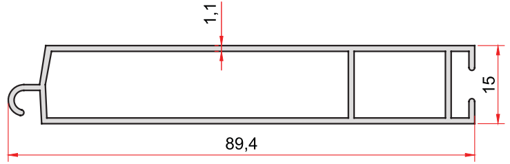
KOD-CODE TEORİK AĞIRLIK THEORETICAL WEIGHT 2302 0,659 Kg/m
