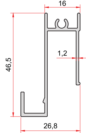
KOD-CODE TEORİK AĞIRLIK 1469 0,413 Kg/m THEORETICAL WEIGHT
