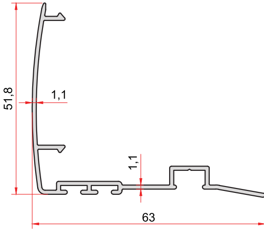
KOD-CODE TEORİK AĞIRLIK KS-4514-11 THEORETICAL WEIGHT 0,448 Kg/m
