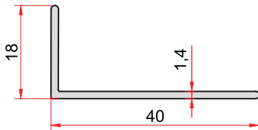
KOD-CODE TEORİK AĞIRLIK THEORETICAL WEIGHT 156 0,211 Kg/m
