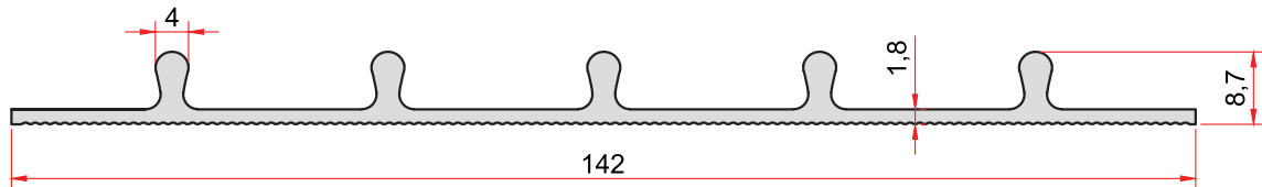
KOD-CODE TEORİK AĞIRLIK THEORETICAL WEIGHT 2384 0,955 Kg/m
