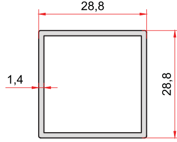
KOD-CODE TEORİK AĞIRLIK THEORETICAL WEIGHT 5083 0,413 Kg/m
